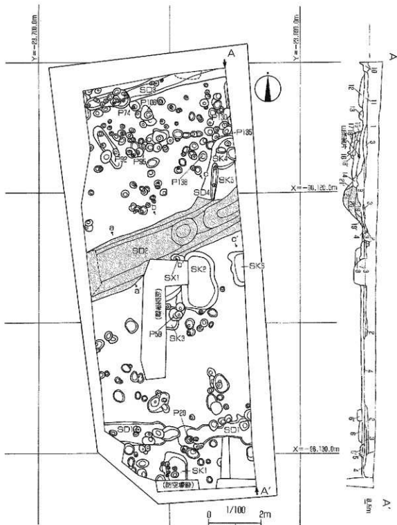
第22図 14次調査遺構平面図および土層断面図 (1/100)
