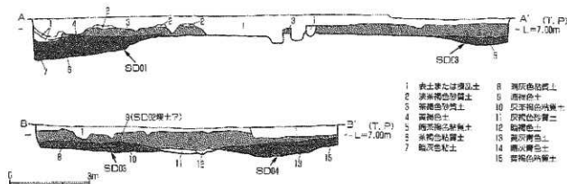
第6図 12次調査区西壁(A-A')・北壁(B-B')土層断面図
