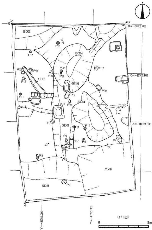
第7图 12次调查区遺構平面图
