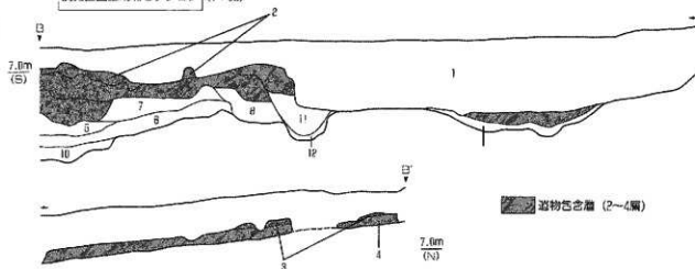
調査区西側南北セクション (1:50)
