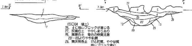
SD04セクション図 (1:50)
