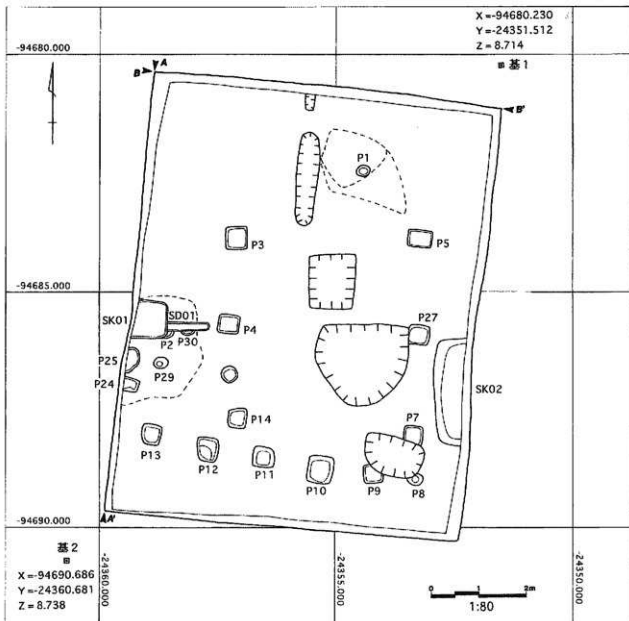
図4 遺構平面図
