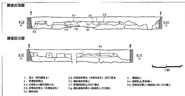
図3 基本土層図
