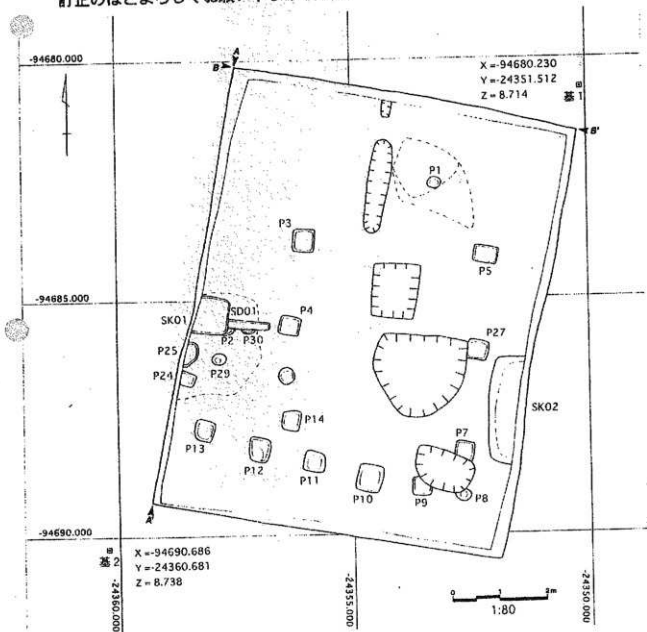
図4 遺構平面図
