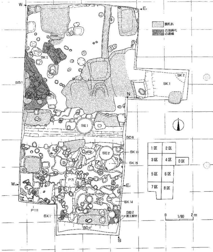
第5図 遺構分布図 (1/80)
