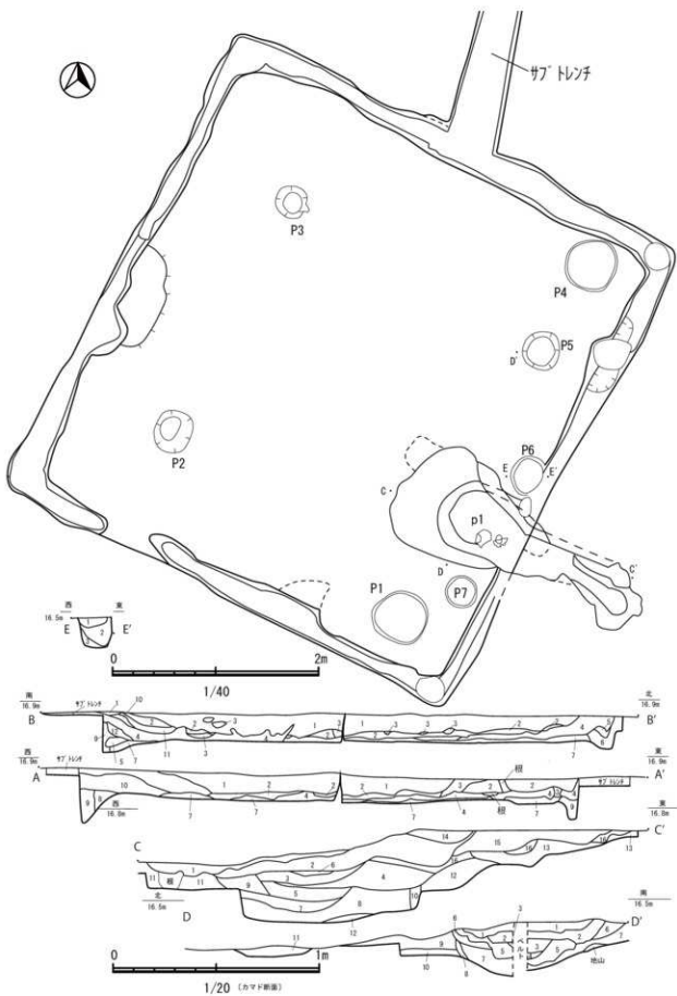
図13 S124下層平面・断面図 (1/40)・カマド断面図 (1/20)
