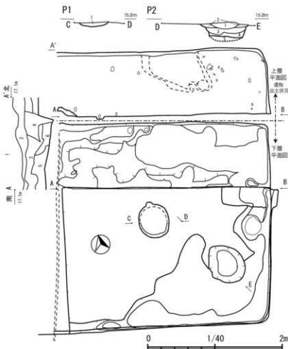
図8 S101平面・断面図 (1/40)
