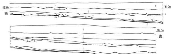
図5 基本層序
