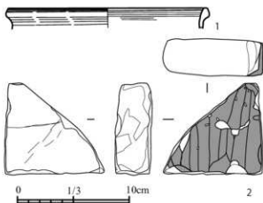
図18 S117・19出土遺物実測図(1/3)
