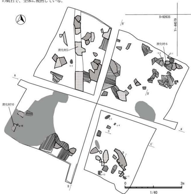
図12 S124炭化材・遺物出土状況実測図(1/40)
