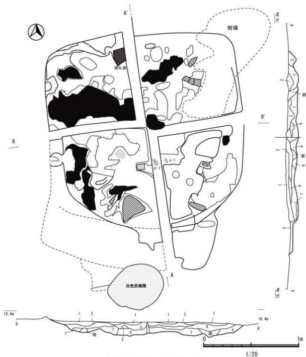
図21 SK21平面・断面図 (1/20)
