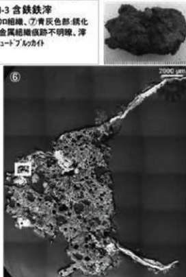
写真116 錬滓・含鉄鉄滓の顕微鏡組織
