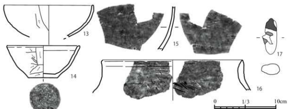
図23 SK出土遺物実測図 その2 (1/3)
