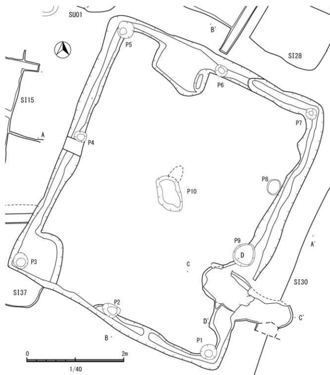
図16 SX16下層・周辺遺構平面図(1/40)
