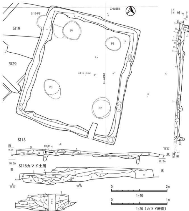
図10 SI18下層・カマド平面・断面図 (1/40) (1/20)
