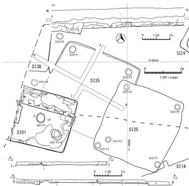
図19 S101・25・35・38平面図(1/60)・断面図(1/40)
