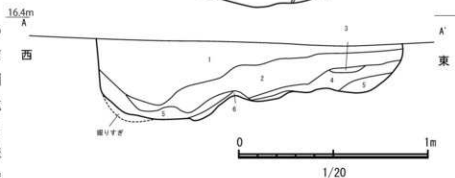
図25 SK23平面・断面図 (1/20)
