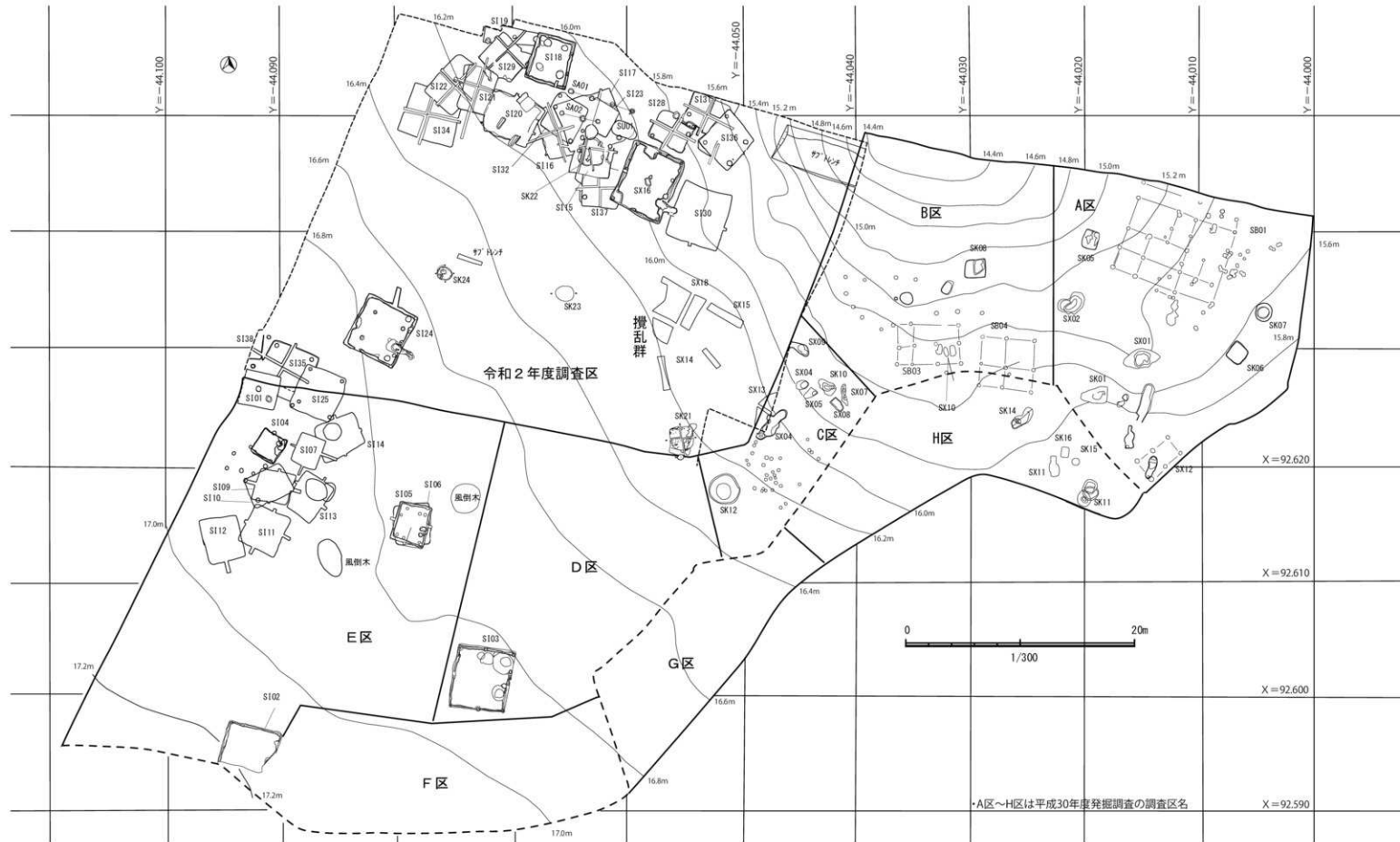
図6 遺構配置図 (1/300)
