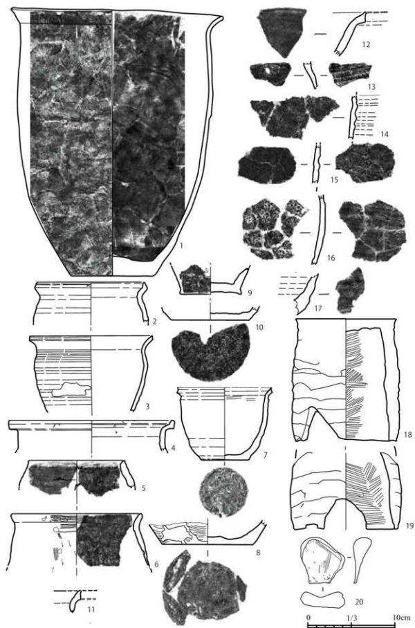
图11 S118出土遺物実測図 (1/3)
