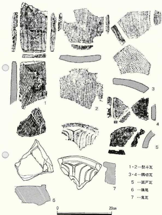
第16圖 出土道具瓦 (1:4)
