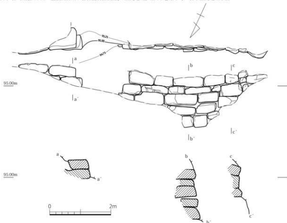
第25図 東石墨実測図 (1/60)
