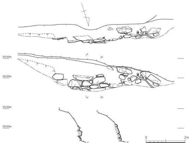
第 23 図 中門南西石壁実測図 (1/60)
