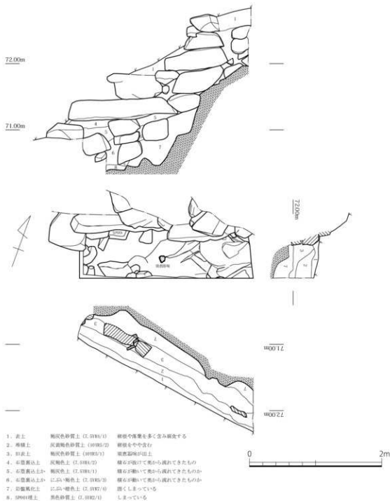
第14図 B5トレンチ実測図 (1/40)
