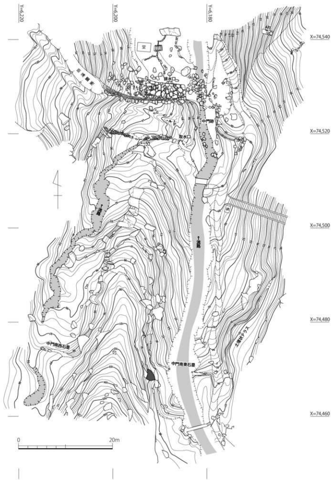
第 21 図 中門跡背面地形測量図 (1/400)
