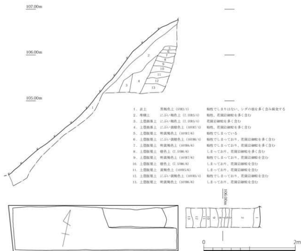
第9図 B3トレンチ実測図 (1/40)
