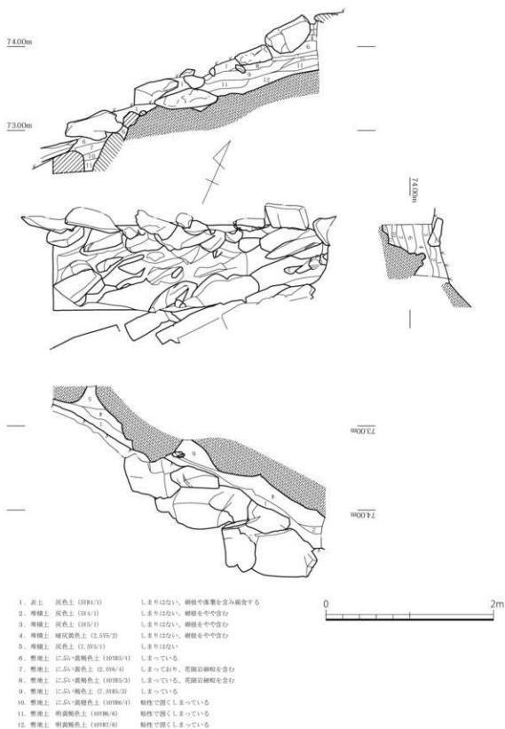
第 13 図 B4 トレンチ実測図 (1/40)
