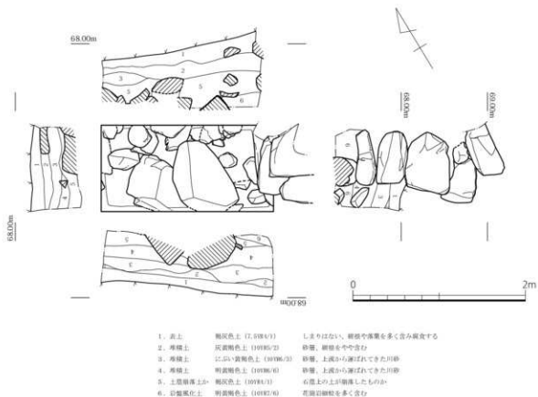
第16図 B6トレンチ実測図 (1/40)
