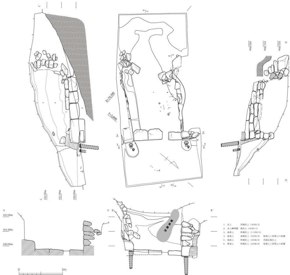
第18図 第2東門跡平面・立面・断面図 (1/80)
