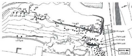
目地の状況・その他(矢穴・刻印等)
