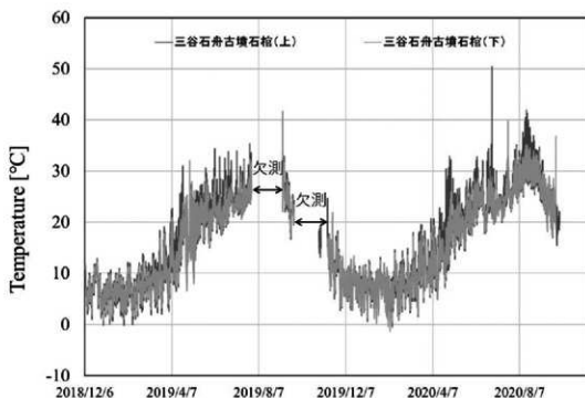
図 41 三谷石舟古墳石棺の表面温度
