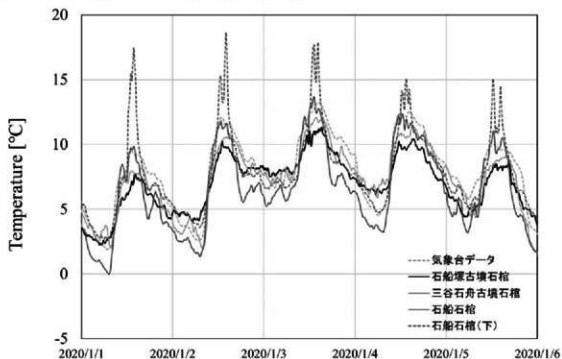
図 27 各石棺周辺の気温 (冬季)
