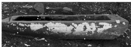
図9 三谷石舟古墳石棺のエコーチップ試験測定箇所（2019年6月実施）
