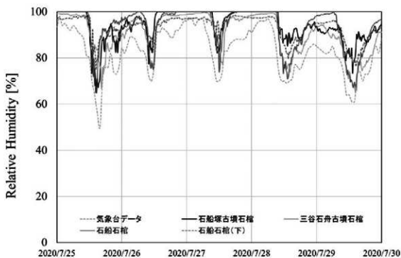
図 34 各石棺周辺の相対湿度 (夏季)
