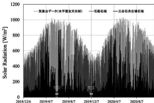
図38 水平面日射量（調査期間全体）
