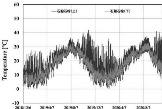
図 42 石船石棺の表面温度
