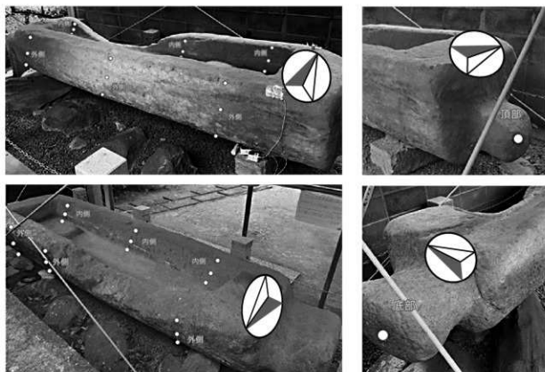
図 22 石船石棺の表面含水率測定箇所（2019 年 9 月）
