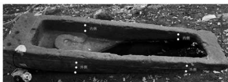
図8 石船塚古墳石棺のエコーチップ試験測定箇所（2019年6月実施）
