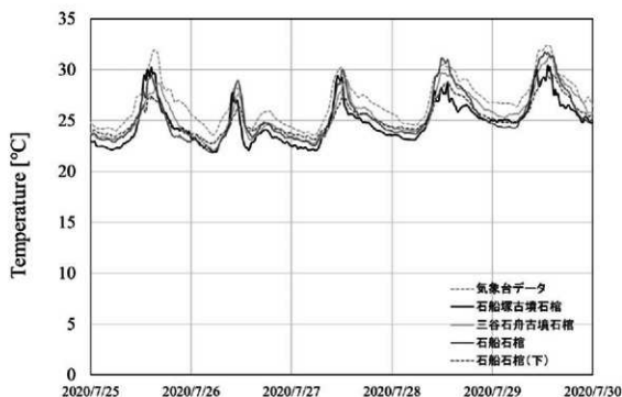
図 28 各石棺周辺の気温 (夏季)
