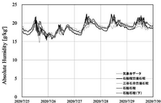
図 31 各石棺周辺の絶対湿度（夏季）
