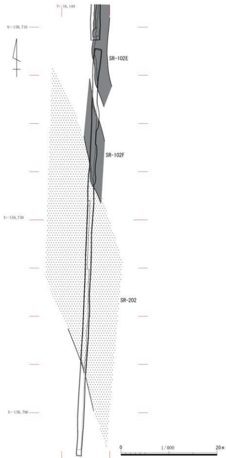
第15図 第2トレンチの遺構 (S=1/400)
