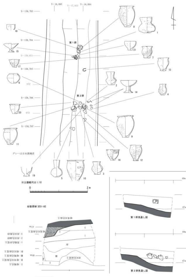
第14図 SR-102E 出土状況と層序(S=1/40)
