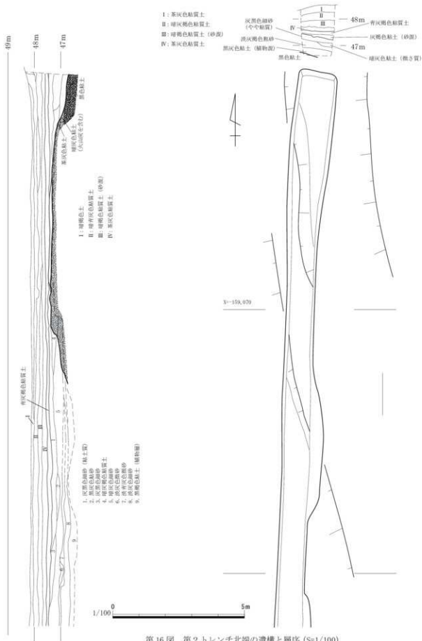
第16図 第2トレンチ北端の遺構と層序 (S=1/100)
