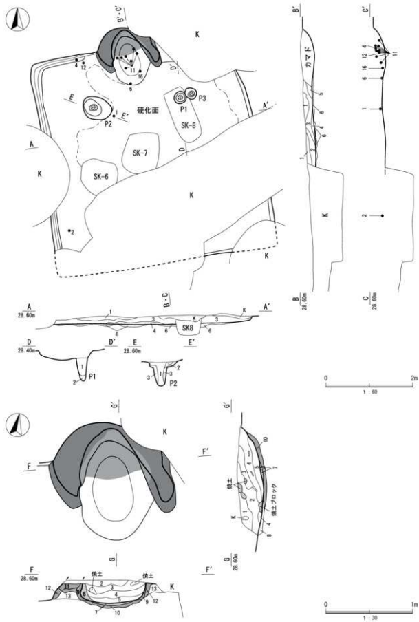
第10図 第2号竖穴建物跡実測図
