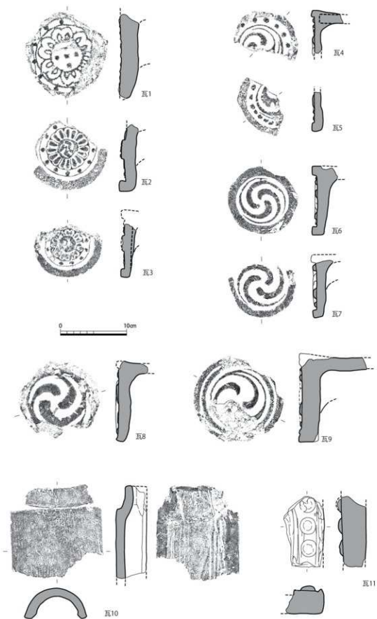
图19 出土瓦类测图(1:4)·拓影1
