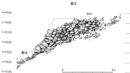
図27 E-C-D間立面概念図（1：100）
