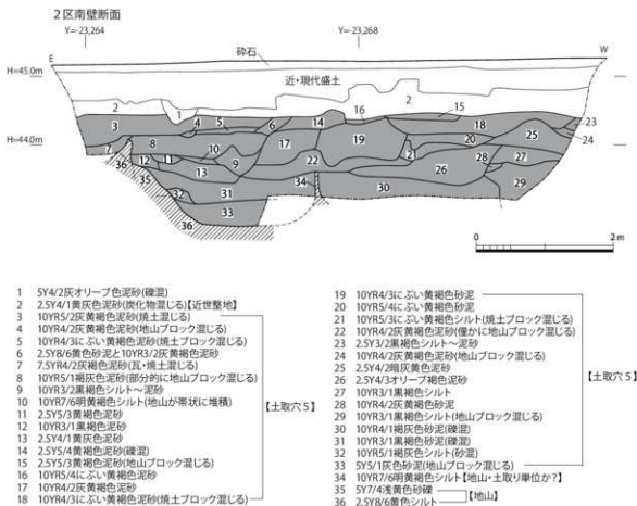
図10 2区南壁断面図(1:60)
