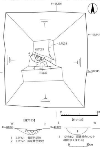
図15 2区第4面平面(1:60)・各遺構断面図(1:30)
