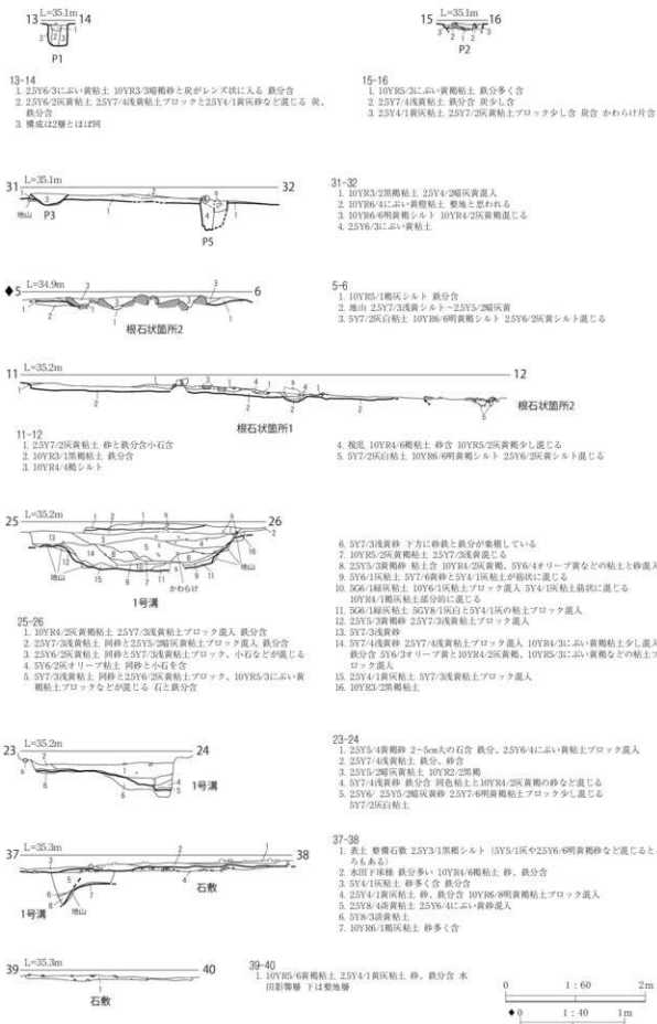
第7図 断面図(1)
