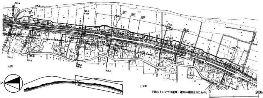
第28図 大野地区トレンチ配置図(S=1/4,000)
