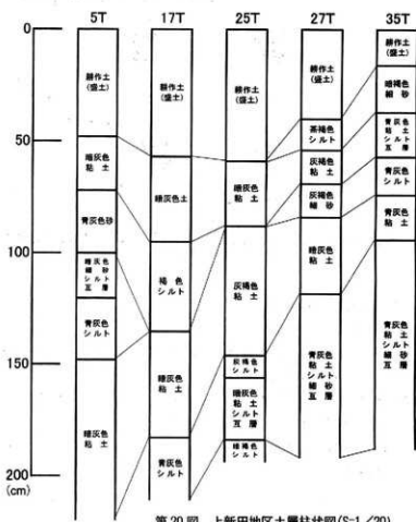
第20図 上新田地区土層柱状図(S=1/20)
