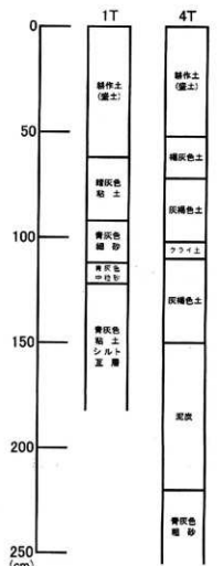
第14図 万年地区土層柱状図(S=1/20)
