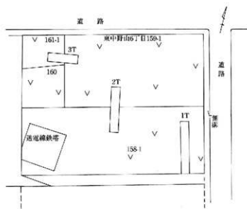
図2 トレンチ配置図 S = 1/500
