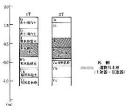
図3 土層柱状図
