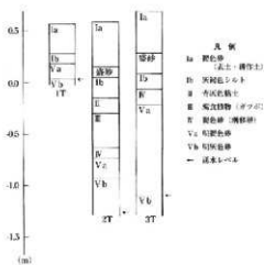
図3 土層柱状図
