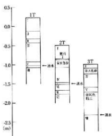
図3 上層柱状図
