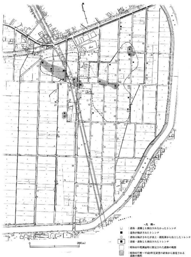
図4 範囲再考図
