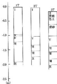
図3 土層柱状図
