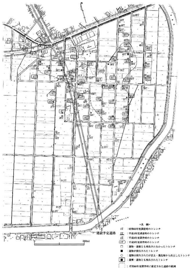
図3 昭和60年～平成9年の調査におけるトレンチ配置図および結果
