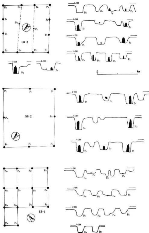
第12図 掘立柱建物柱穴断面図
