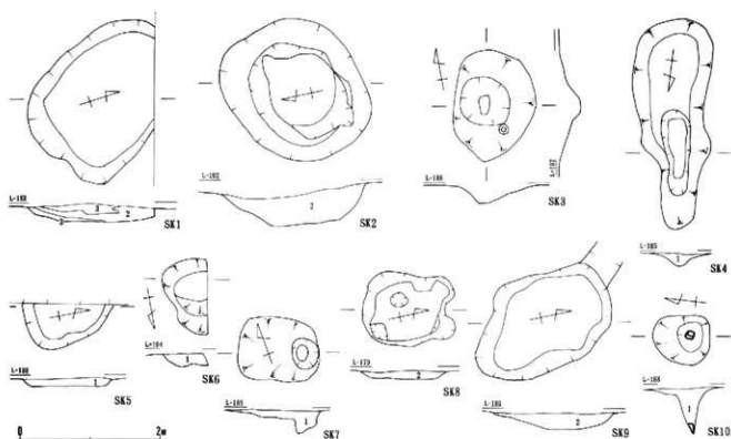
第30図 土坑平断面図
