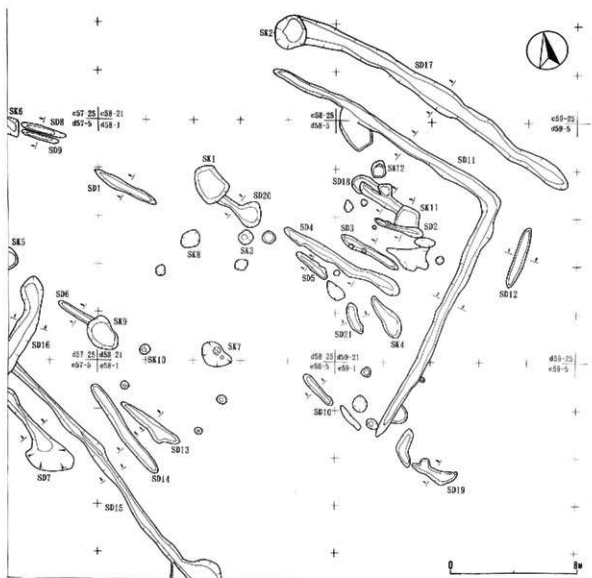
第28図 遺構全測図
