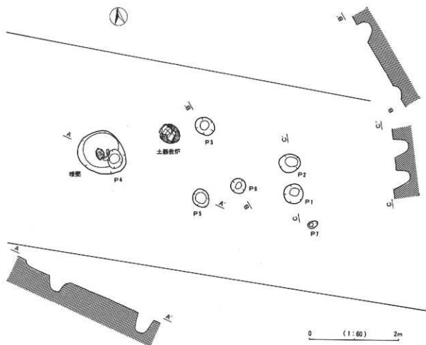
第38図 J3号住居址実測図
