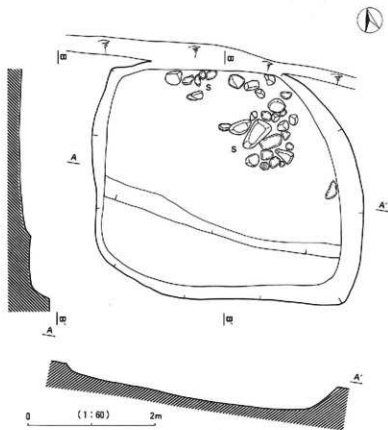
第14図 T1号特殊遺構実測図No.2
