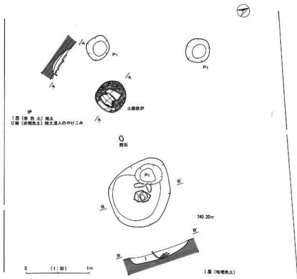
第39図 J3号住居址・埋藏実測図
