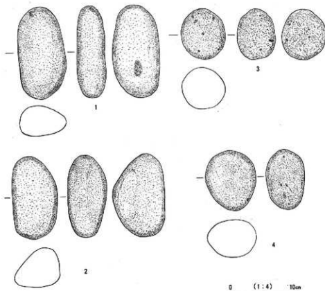
第16図 T1号特殊遺構出土石器実測図
