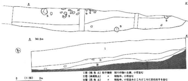
第30図 溝状遺構実測図
