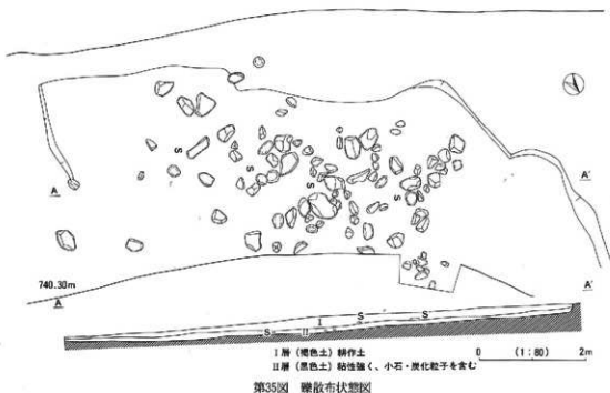
第35図 礫散布状態図
