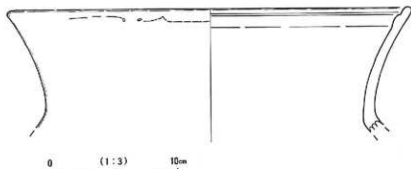
第36図 調査区外出土土器実測図
