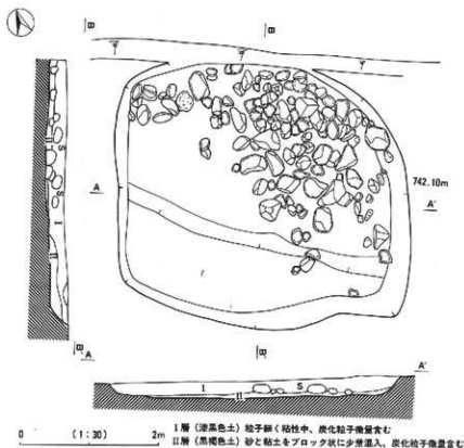
第13図 T1号特殊遺構実測図
