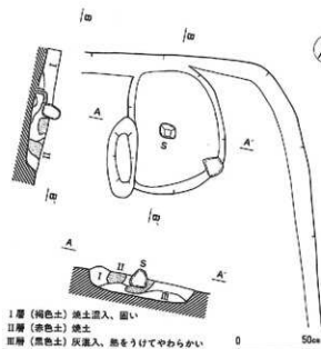
第23図 H1号住居址カマド実測図
