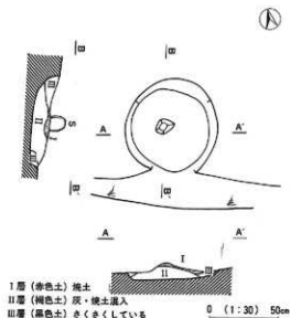
第24図 H1号住居址灰溜実測図
