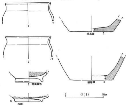
第25図 H1号住居址出土土器実測図
