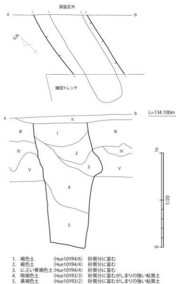
1号土坑 (SC1・隠し穴状遺構) 実測図
