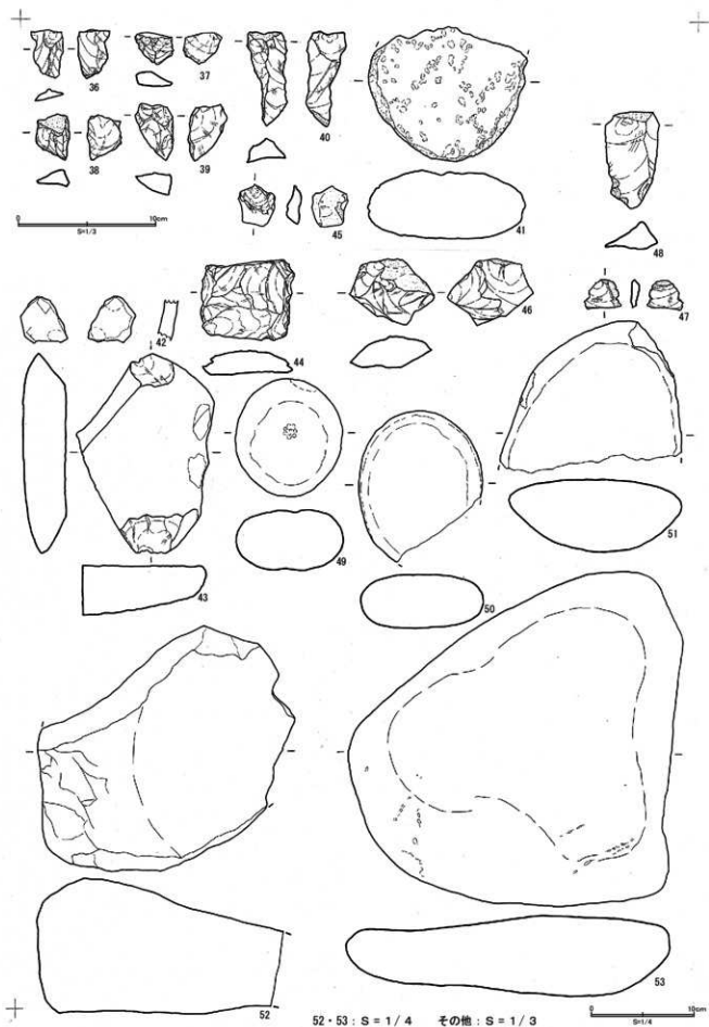
第 17 図 縄文時代早期 遺物実測図 (2) (36 ~ 41 : VI層下位、42 ~ 53 : VII層)
