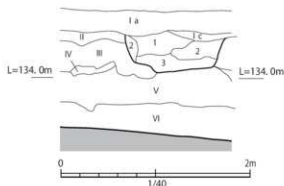
3号土坑 (SC3) 実測図
