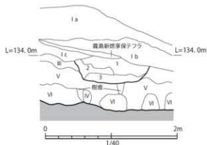
2号土坑 (SC2) 実測図
