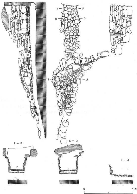
第4图 真光寺第1号古墳石室及び前庭部実測図(1:80)
