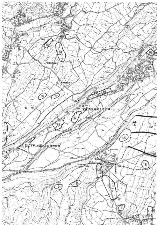
第1図 真光寺第1号古墳位置図及び周辺道跡分布図 (1:10,000)
