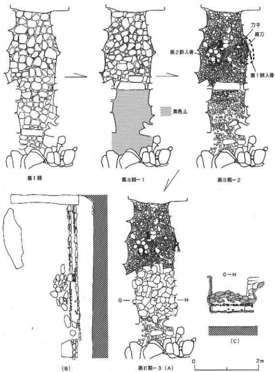
第5图 真光寺第1号古墳石室構築及び倒塌状態 (1:60)
