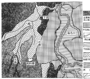
第3図 浅科村地形分類図
