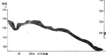
第5図 矢嶋城A-B断面
