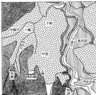
第8図 浅料村地質図
