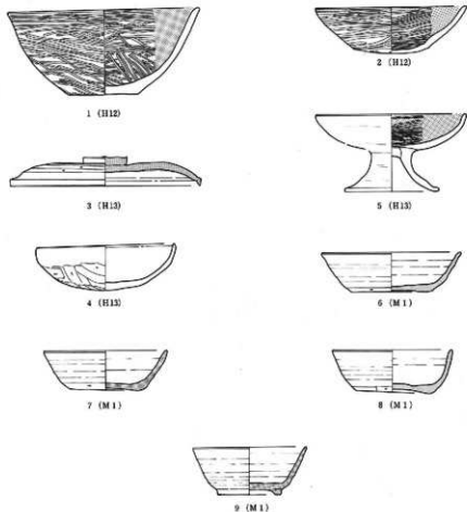
第15図 H12号・H13号住居址・M1号溝状遺構出土遺物実測図
