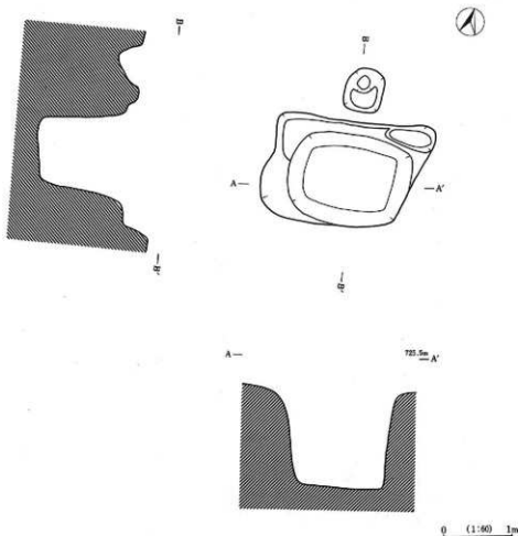
第6図 H5号住居址貯蔵穴実測図
