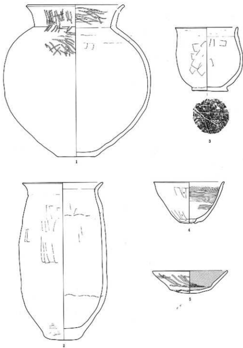
第14图 H11号住居址出土遺物実測図
