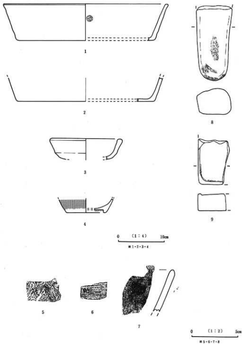
第9图 新町遗址出土文物实测图·拓影图
