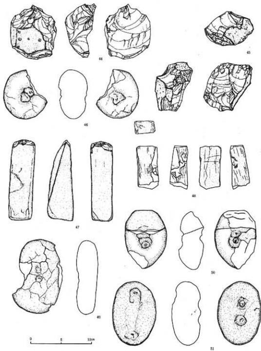
第8图 五斗代B遗址出土石器实测图(1:3)
