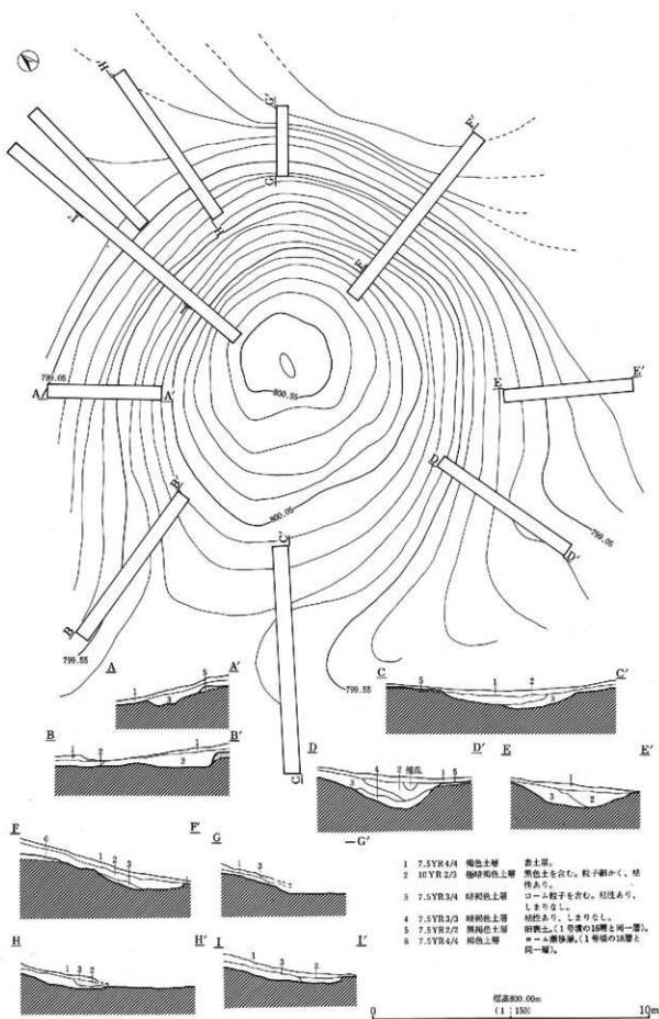
第13図 瀬の峯2号墳墳丘測量図及びトレンチ設定図
