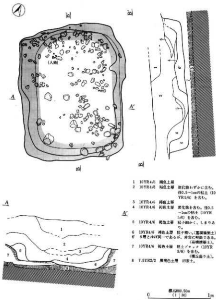
第17図 瀬の峯2号墳墓墳実測図
