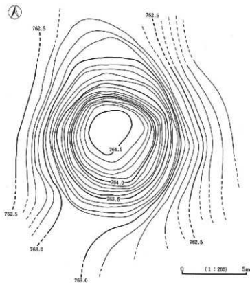
第21図 瀬の峯5号墳丘陵測量図
