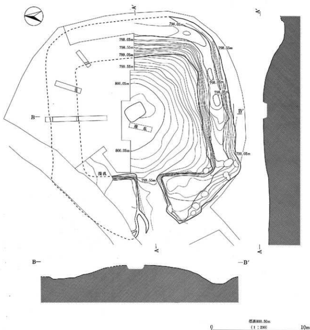
第14図 麓の峯2号墳平面図
