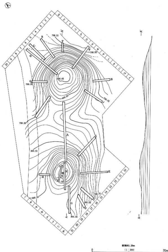
第7図 瀬の峯1・2号墳丘陵測量図及びトレンチ設定図
