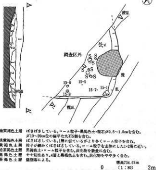
第13図 第3号住居址実測図
