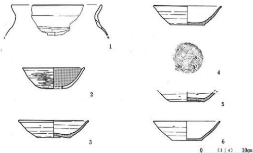
第21図 第1号特殊遺構出土土器実測図
