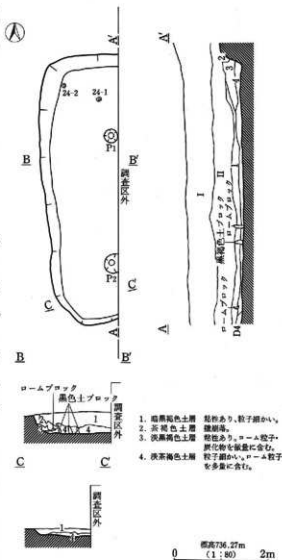
第23図 第1号竪穴状遺構実測図
