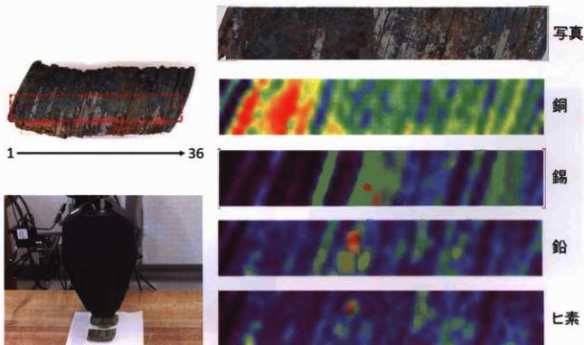
図10 蛍光X線分析による「さし銭」の元素マッピング
