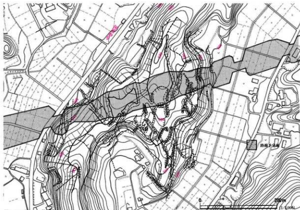
図12 中根館跡概略図
