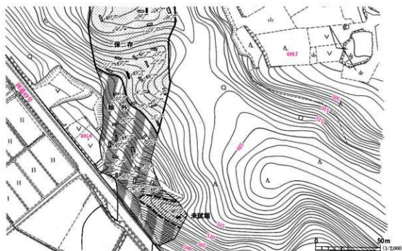
図14 中根館跡トレンチ配置図(2)
