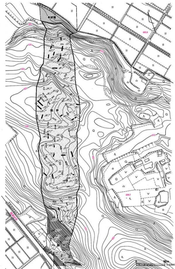
図13 中根館跡トレンチ配置図(1)
