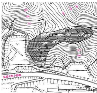
図9 ON-B6トレンチ配置図
