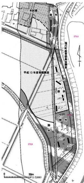
図61 荒屋敷遺跡トレンチ配置図
