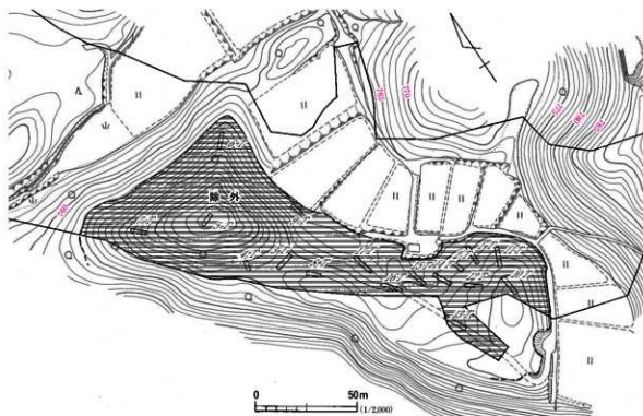
図70 CG-B4トレンチ配置図
