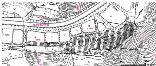
図19 HT-B1トレンチ配置図
