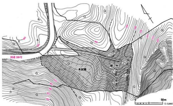
図72 CG-B6トレンチ配置図
