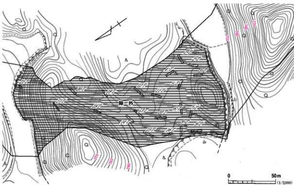
図69 CG-B3トレンチ配置図
