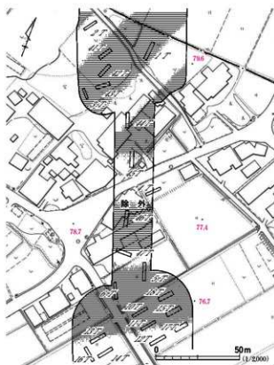
図44 大石原遺跡トレンチ配置図
