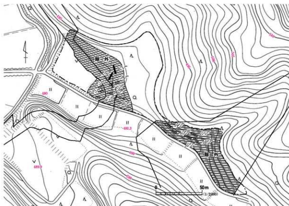
図31 B12トレンチ配置図
