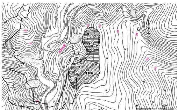
図39 B7トレンチ配置図
