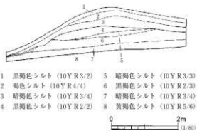
図15 63号トレンチ断面図
