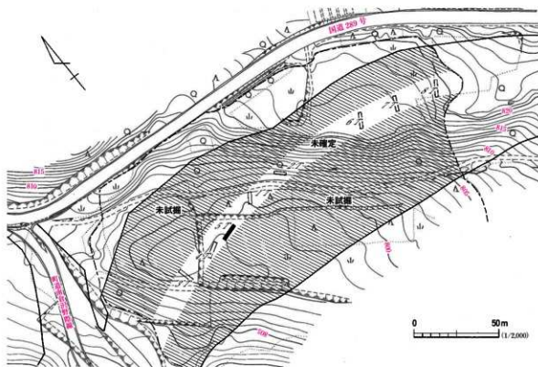
図71 CG-B5トレンチ配置図
