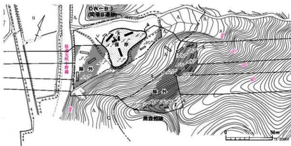
図5 黒森館跡・ON-B3（開場B遺跡）トレンチ配置図
