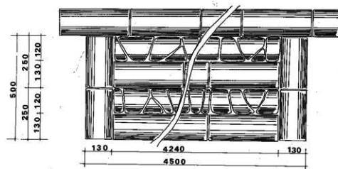
階段断面図
