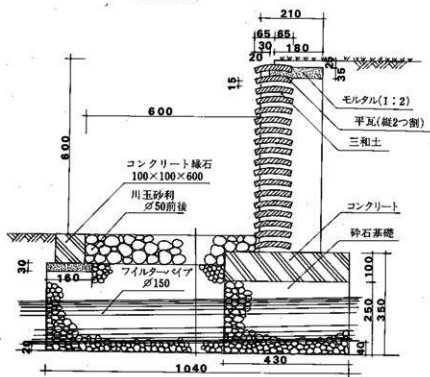
基礎断面図
