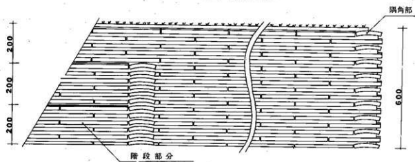
基礎・階段正面図
