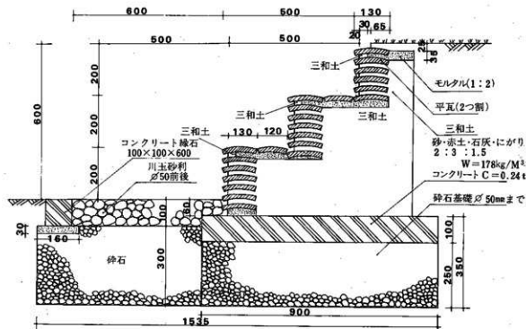
第10図 講堂跡基礎復原計画部分詳細図
