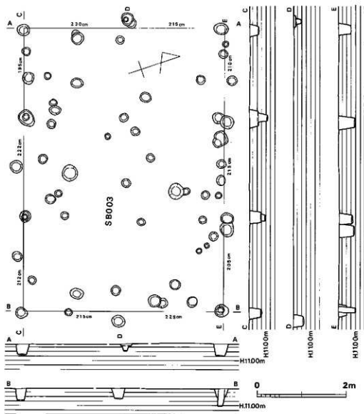
第7図 3号掘立柱建築物(縮尺1/60)
