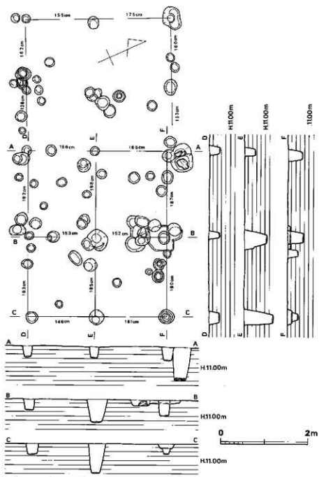
第 6 图 2 号架立柱建筑物 (缩尺 1/60)
