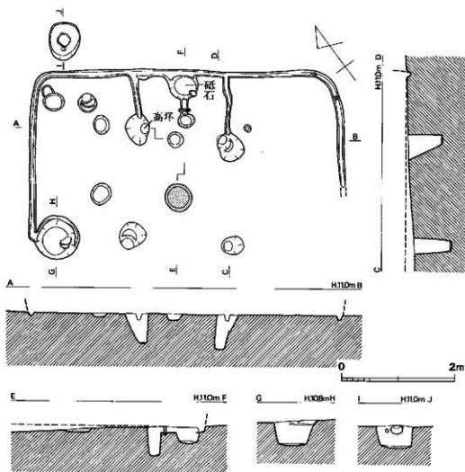
第 11 図 D 地点聚穴住居跡実測図 (縮尺1/60)
