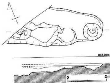
第15図 D地点溝状遺構(縮尺1/60)
