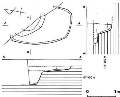
第8図 1号土坑 (縮尺1/40)
