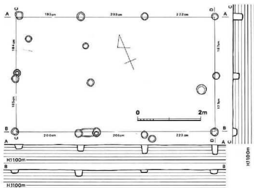
第5図 1号掘立柱建物(縮尺1/60)
