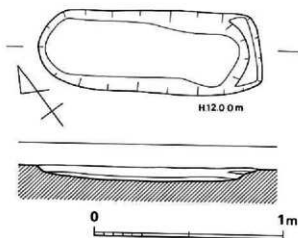
第 14 図 D地区土塚実測図 (縮尺1/20)
