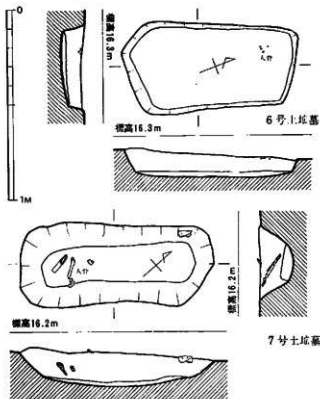
第71図 6・7号土塚墓実測図 (1/20)
