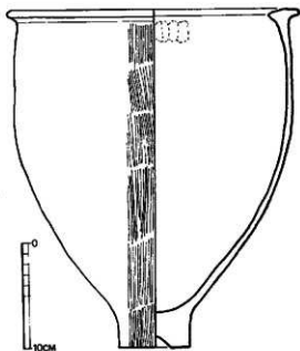
第 44 図 住居跡内出土遺物実測図① (1/4)
