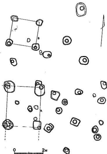
第82図 掘立柱穴遺構実測図 (1/80)
