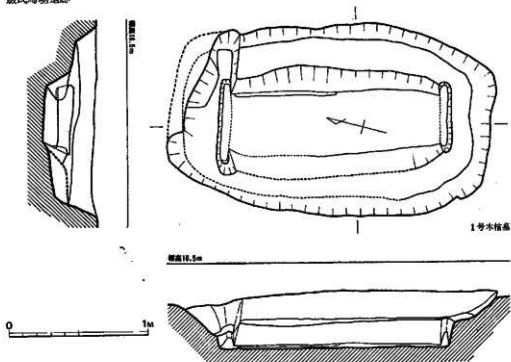
第48图 1号木棺基实例图 (1/20)
