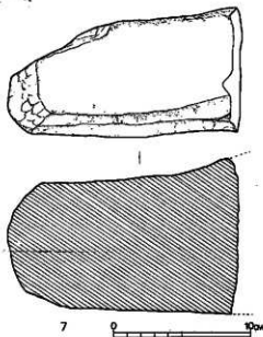
第49図 住居跡床面出土遺物実測図(1/3)
