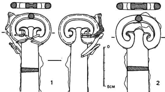
第21図 鉄製環頭大刀部分実測図(2/3)
