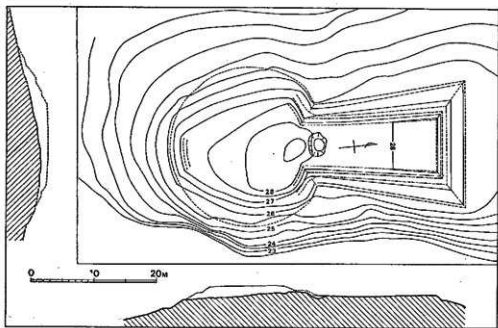
第 30 圖 若八幡宮古墳地山削土圖 (1/600)
