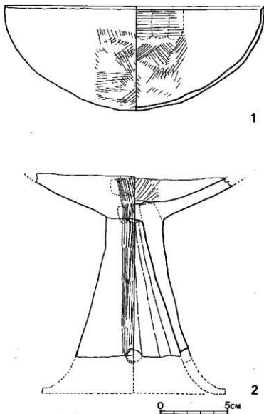
第72図 pit 遺構出土遺物実測図 (1/2)
