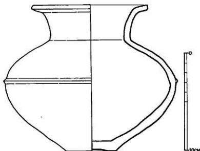
第45図 住居跡内出土遺物実測図㊸ (1/2)
