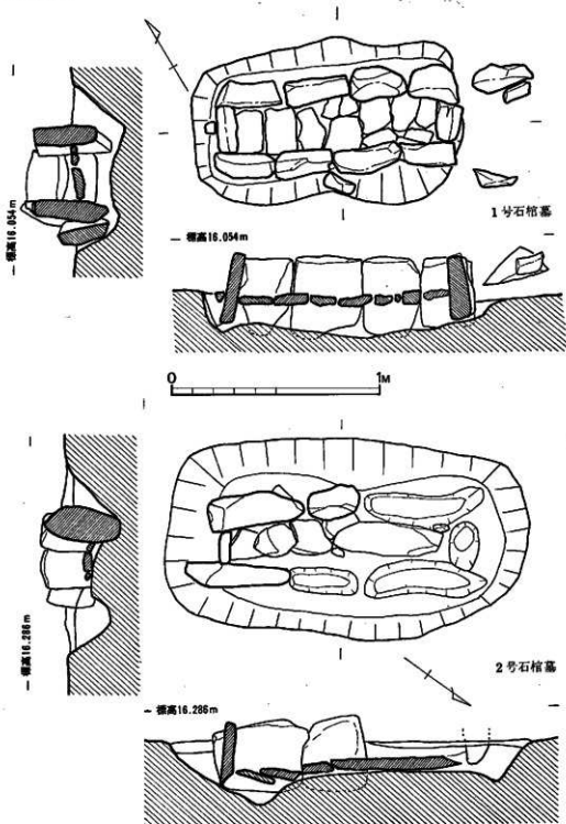
第55图 1・2号石棺墓平面剖面图
