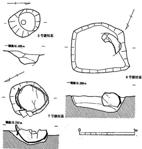
第 58 図 5・6・7 号壺棺墓実測図 (1/20)
