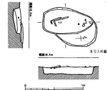
第 89 図 4・5号土塚墓実測図 (1/20)
