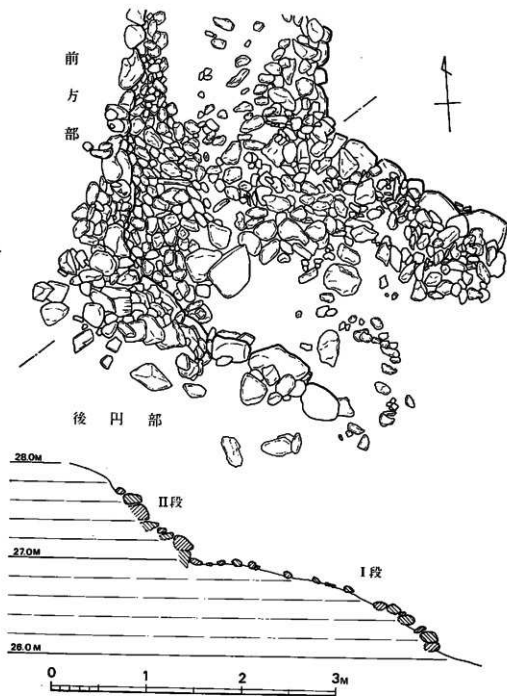
第11図 東側くびれ部葺石実測図 (1/40)
