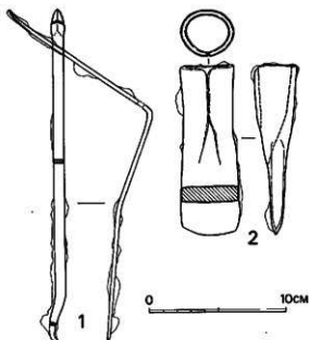
第24図 鉄施・鉄弁実測図 (1/3)
