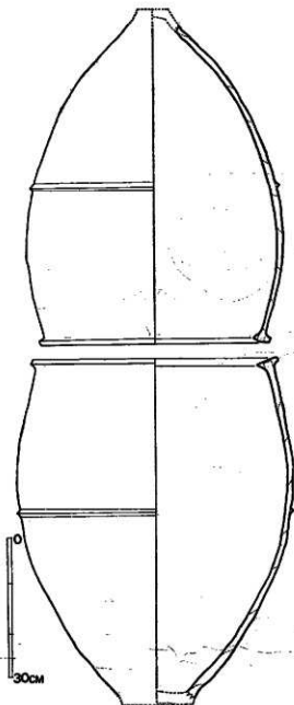
第54図 4号甕棺実測図 (1/9)
