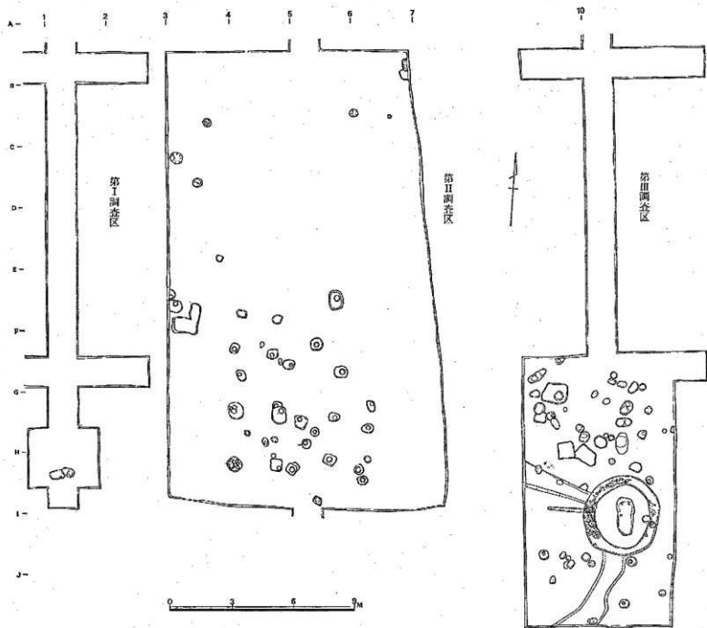
第 19 圖 遺構配置図 (1/100)
