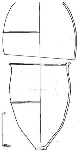
第 55 図 3 号 甕 輪 突 測 図 (1/9)
