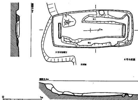
第50図 4号木棺墓実測図 (1/20)
