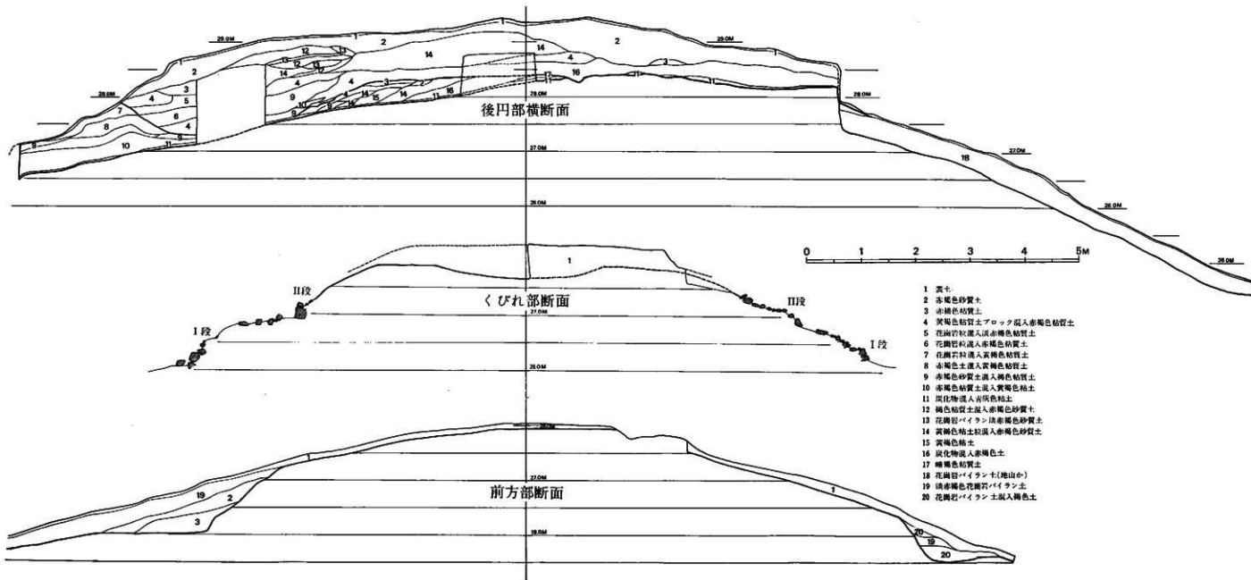
第9図 塚 丘 横 断 面 図 (1/60)
