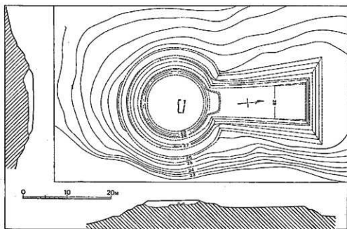
第32図 若八幡宮古墳復原図 (1/600)
