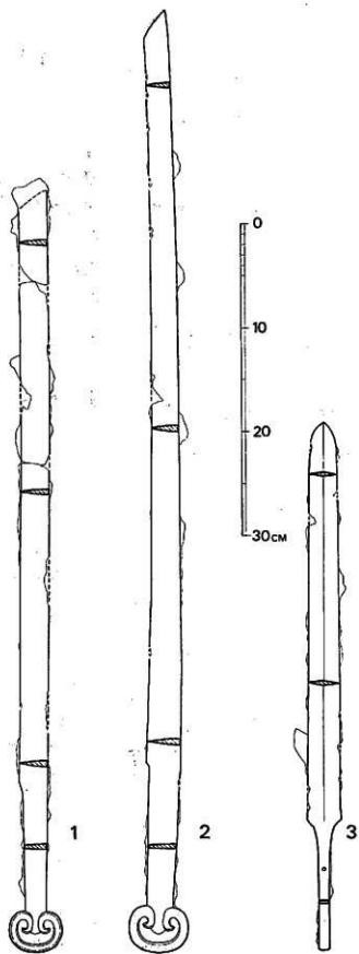
第 20 图 铁製環頭大刀・铁刺实际图 (1/4)
