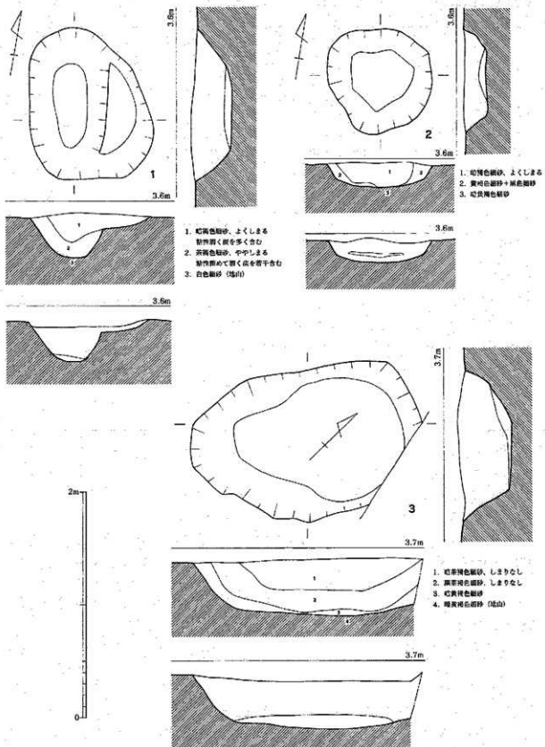
第67図 1～3号土坑実測図 (1/30)
