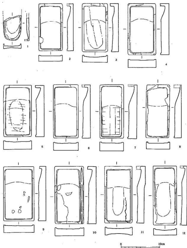
第98图 铜网筛 (1/3)
