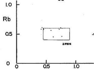
第102図 第13次調査区出土在地系土器の両分布図
