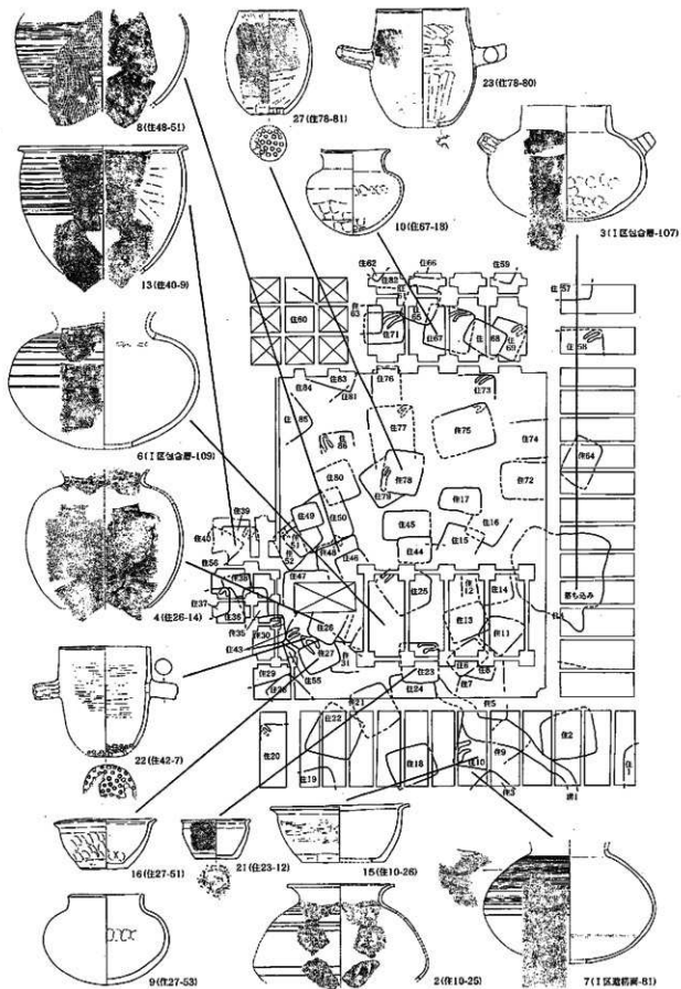
第118图 西新町迹跡第13次調査区出土半島系土器分布图
