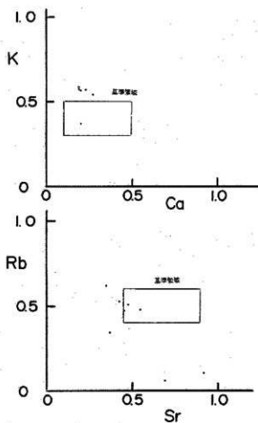
第108図 第12次調査区出土山陰系・吉備系・庄内系土器の両分布図
