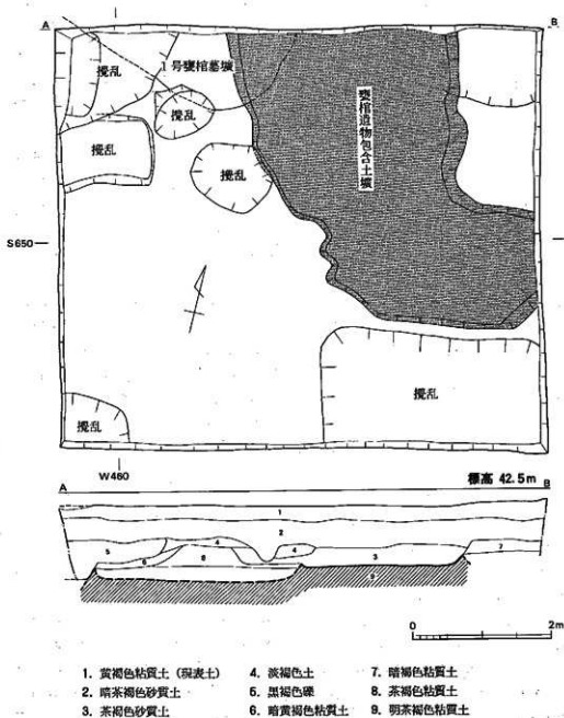
第 4 圖 Ⅰ-6 昭和49年度調査区と北壁土層図 (1/60)
