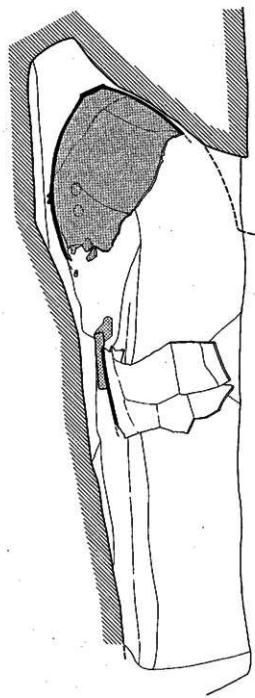
第 26 図 南小路 2 号塚棺墓実測図 (1/20)
