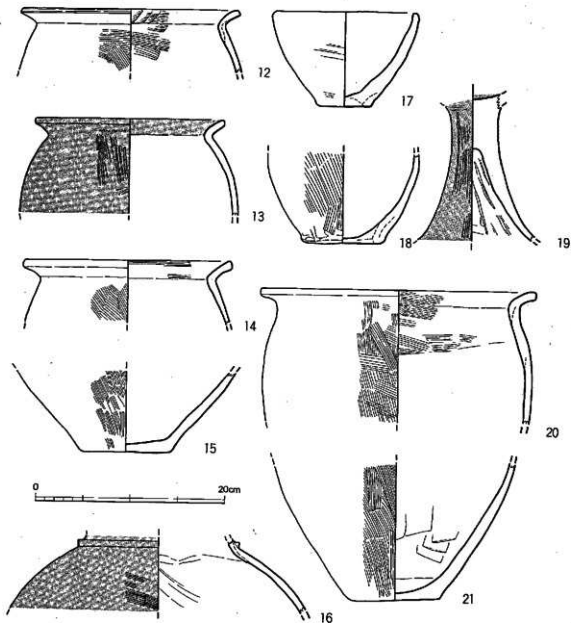
第 39 圖 奈紀溝出土土器実測図③ (1/4)
