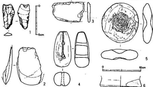
第47図 I-6・7 出土石器類実測図 (1/2・1/3)
