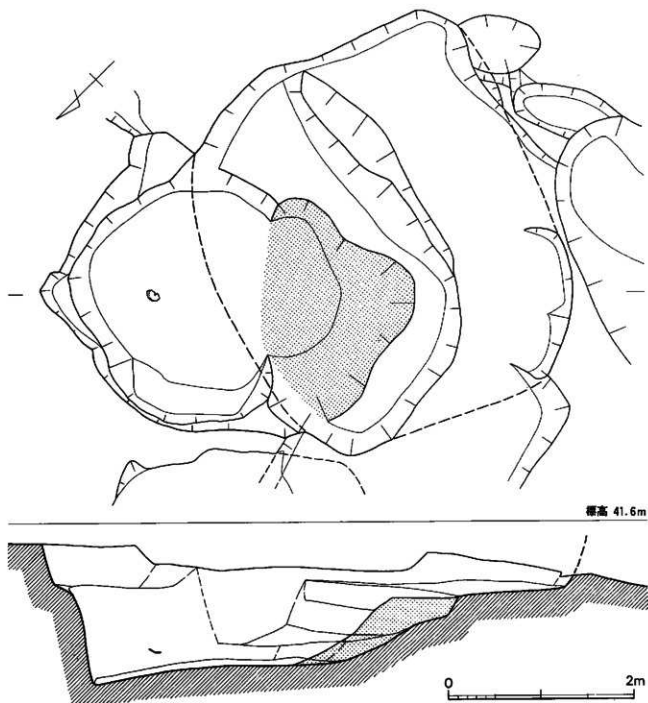
第 6 圖 南小路 1 号雙棺墓實測圖 (1/40)
