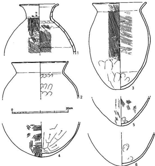
第58圖 I-1・2 出土土器実測図(1/4)
