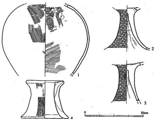
第42図 大溝出土土器実測図 (1/4)
