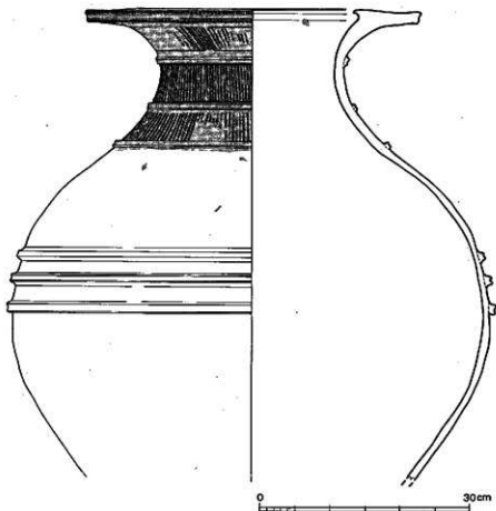
第38図 祭籠溝下層出土土器実測図⑧ (1/6)
