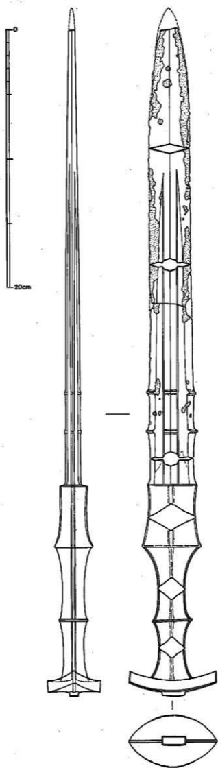
第 8 图 1 号甗坑出土有柄中细刻刺尖测图 (1/2)
