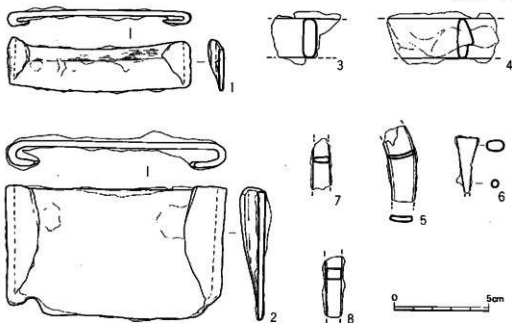
第56図 I-9 山上鉄器実測図 (1/2)
