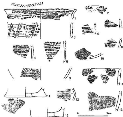
第46図 1-6・7 出土縄文土器実測図 (1/3)
