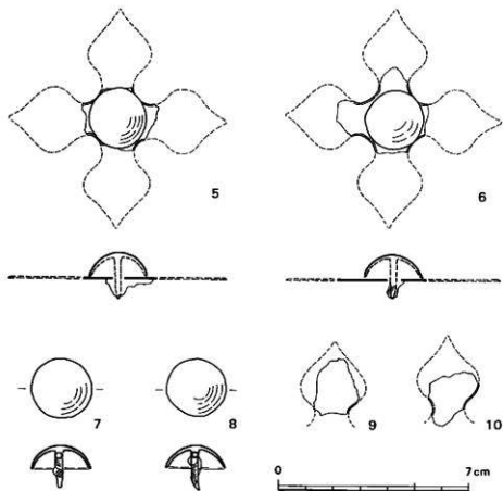
第24図 金銅四葉座飾金具実測図③ (2/3)
