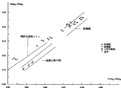
第 59 図 鉛同位体対比プロット図
