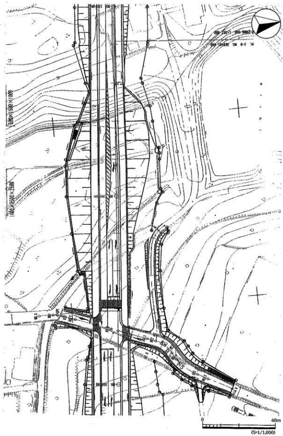
第2図 調査地周辺工事計画図
