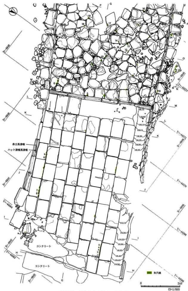
第 12 図 吐井手 (下流側) 平面図①
