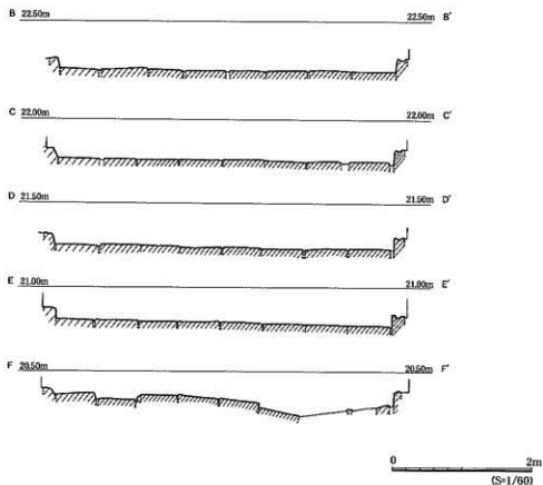
第 11 図 吐井手（上流側）断面図②
