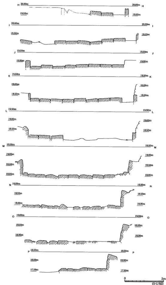
第 16 図 吐井手 (下流側) 断面図③
