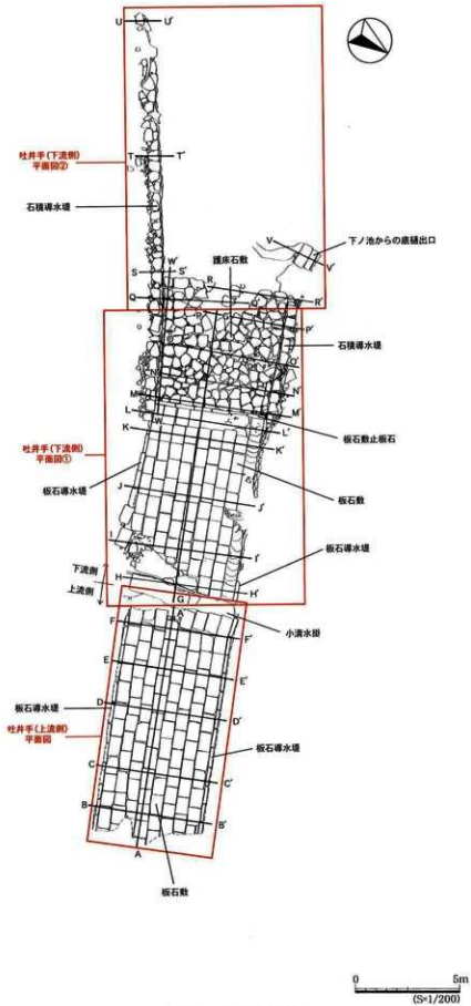
第8図 吐井手全体図
