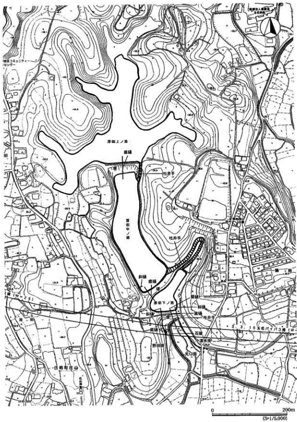
第5図 浮田溜池関連施設配置図
