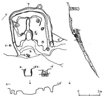
第7図 坂ノ上E遺跡製鉄炉
