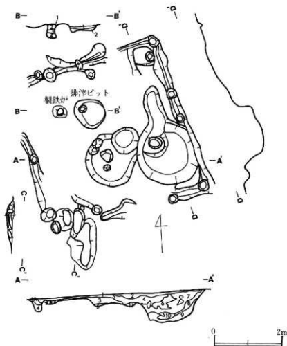
第5図 竹生遺跡製鉄炉
