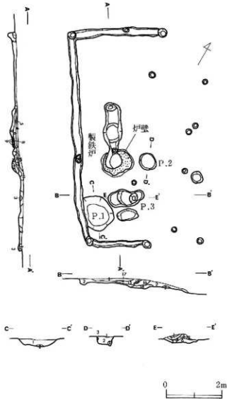
第3図 白長根館I遺跡製鉄炉
