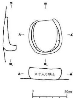
第4図 中台遺跡製鉄炉
