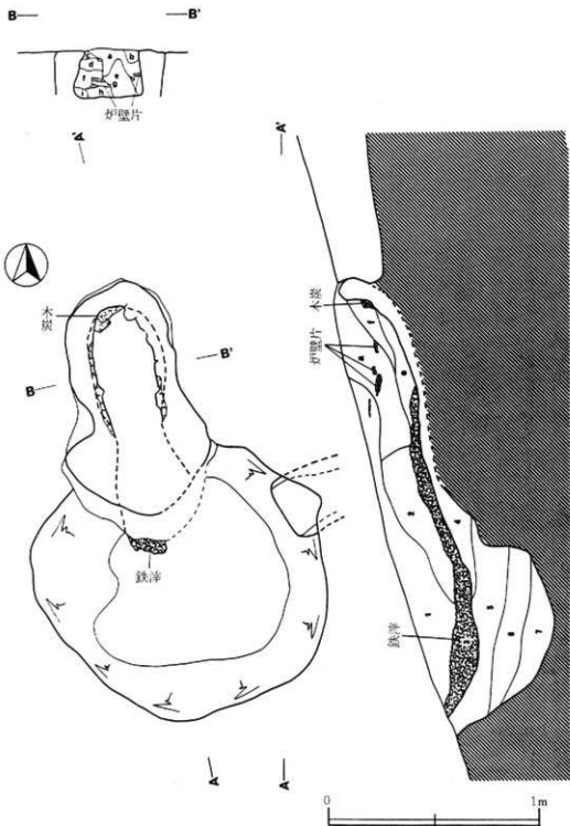
第6図 寒川II遺跡製鉄炉
