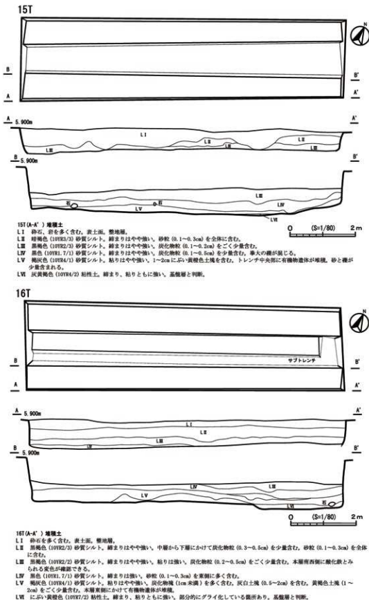
図38 15T・16T平面図・断面図
