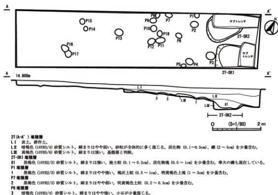
図35 2T平面図・断面図
