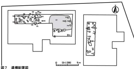
図7 遺構配置図
