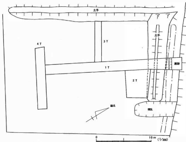
図12 桜井原遺跡トレンチ配置図
