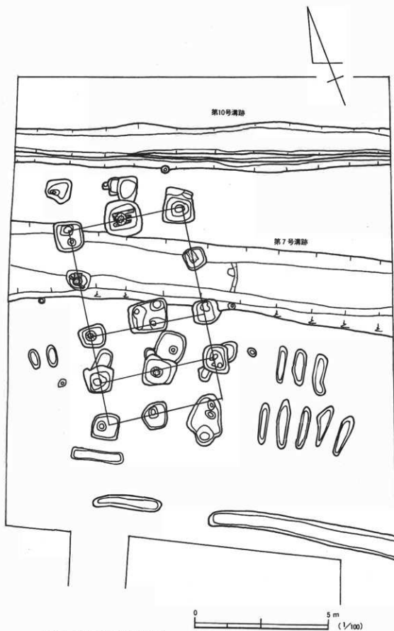
図10 第15号掘立柱建物跡
