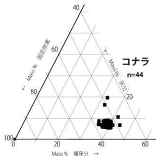
長湍・大船迫A遺跡出土の木炭3成分（固定炭素・揮発分・灰分）の分布図
