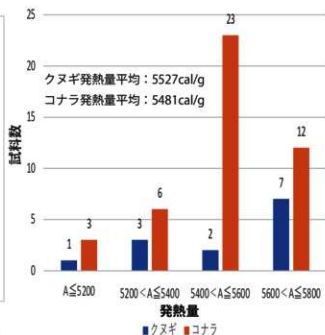
木炭発熱量の平均とヒストグラム
