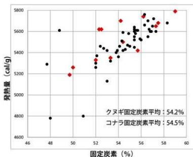
長湍・大船迫A遺跡出土の木炭発熱量と固定炭素の関係
