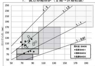
3. 長方形箱形炉 (Ⅳ～Ⅵ期：踏みふいごなし)
