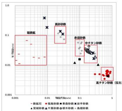
砂鉄の TiO 2 /T.Fe と V/TiO 2 の関係
