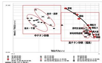
砂鉄の TiO 2 /T.Fe と MnO/TiO 2 の関係
