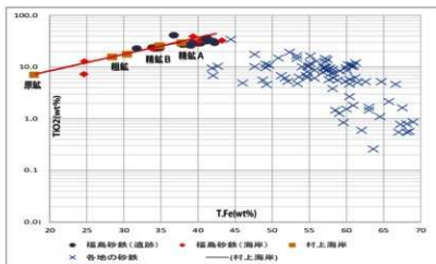
砂鉄の T.Fe と TiO 2 の関係
