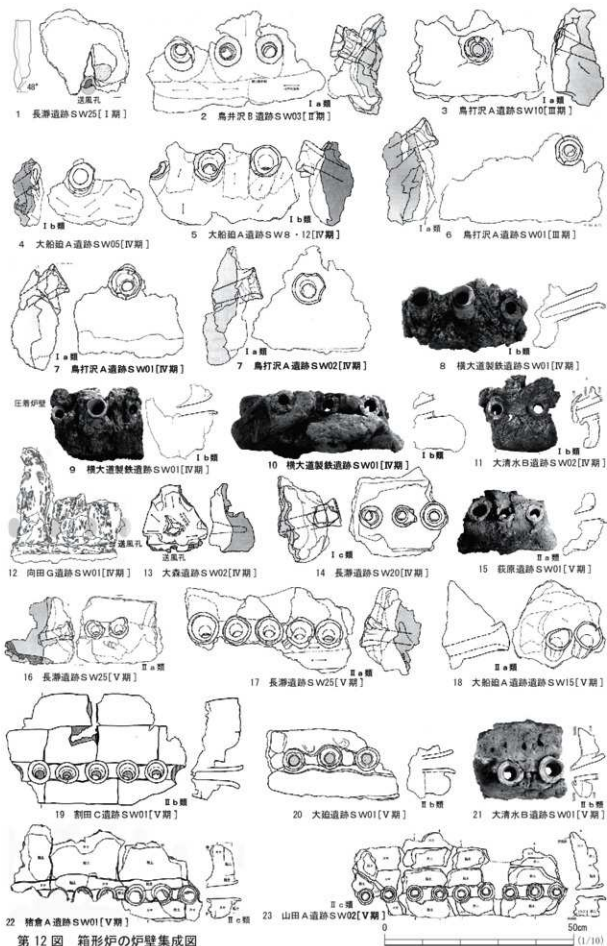
第 12 図 箱形炉の炉壁集成図
