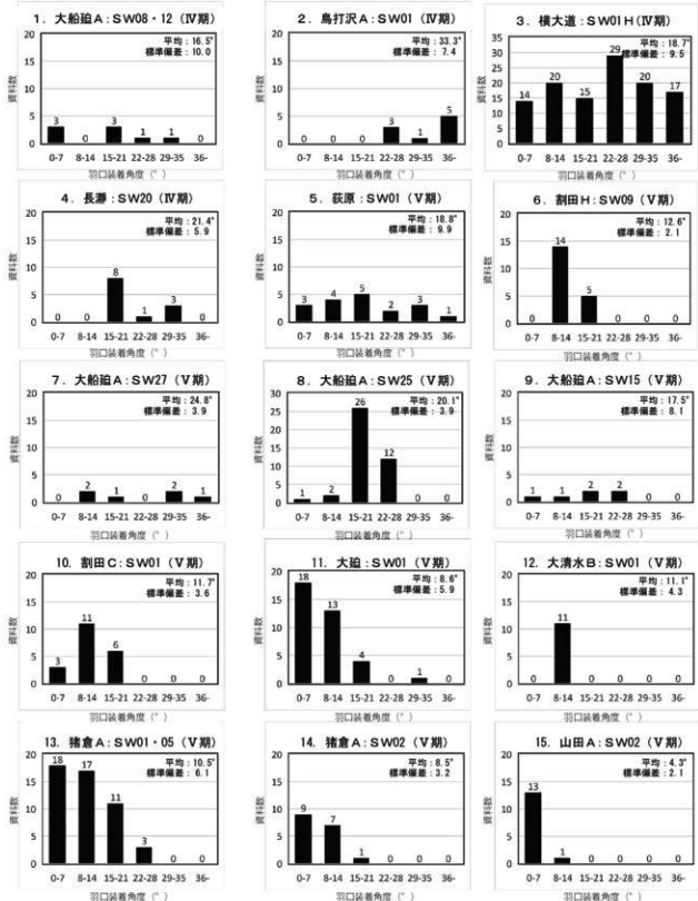
第10図 羽口装着角度の分布
