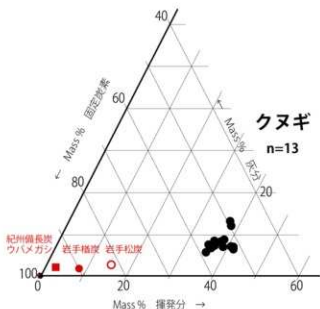
長湍・大船迫A遺跡出土の木炭3成分（固定炭素・揮発分・灰分）の分布図
