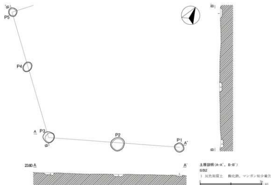
第6図 北島遺跡第2号掘立柱建物跡
