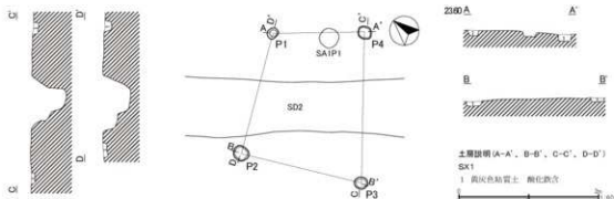
第13図 北島遺跡第1号性格不明遺構
