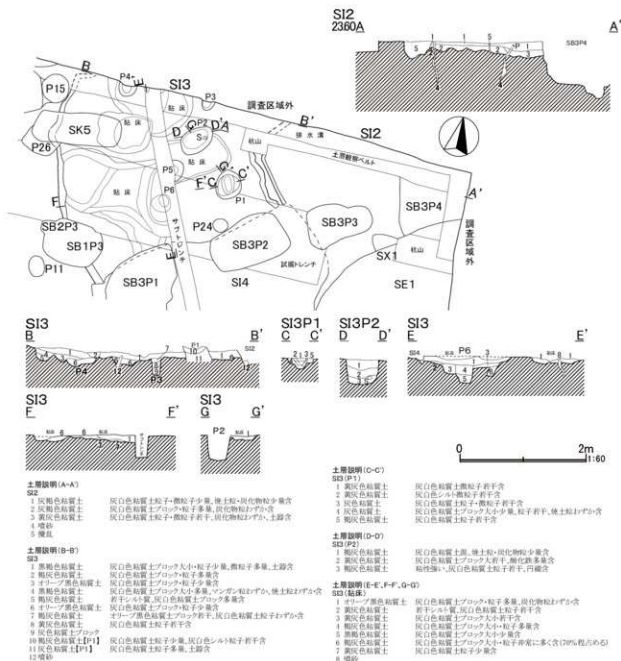
第28図 諏訪木遺跡第2・3号竪穴建物跡
