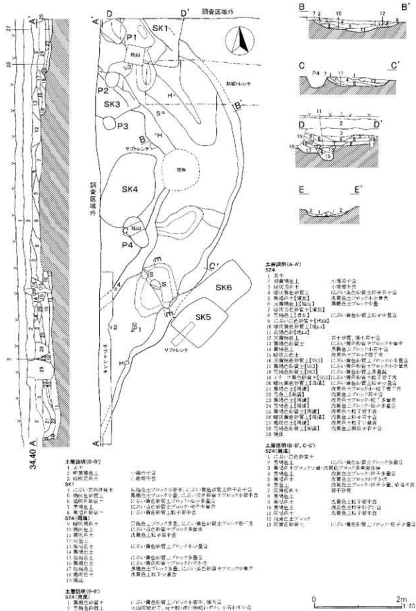
第17図 石原古墳群第4号墳
