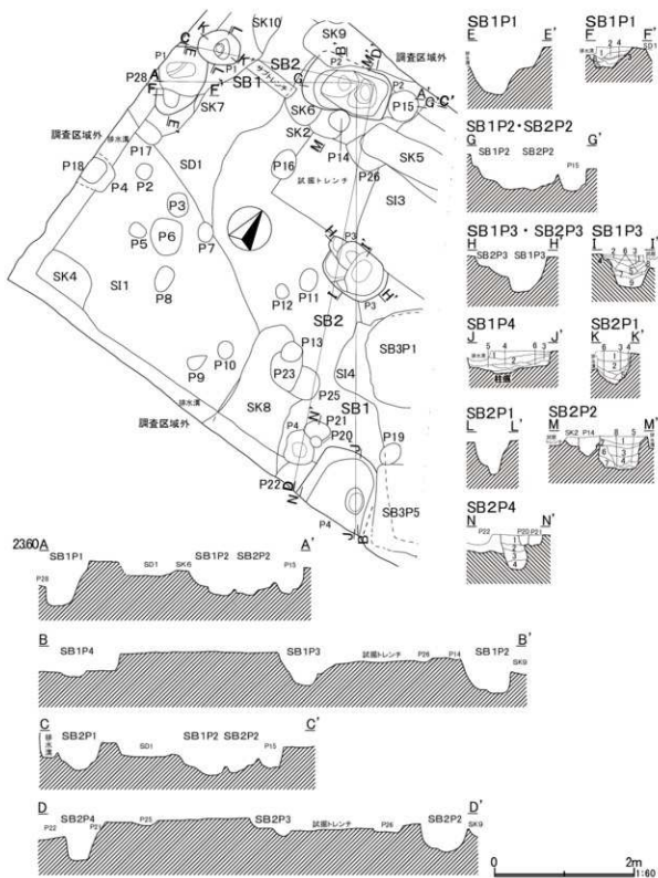
第33図 諏訪木遺跡第1・2号掘立柱建物跡
