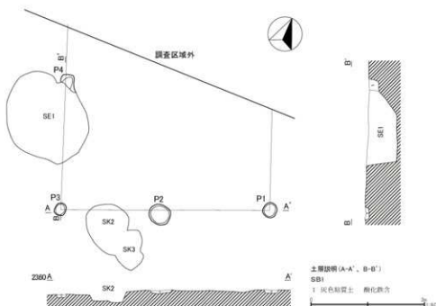
第5図 北島遺跡第1号掘立柱建物跡
