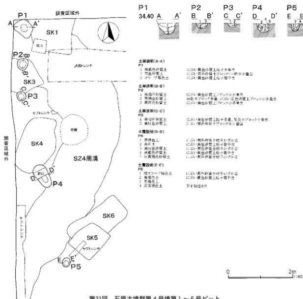
第21図 石原古墳群第4号墳第1～5号ピット
