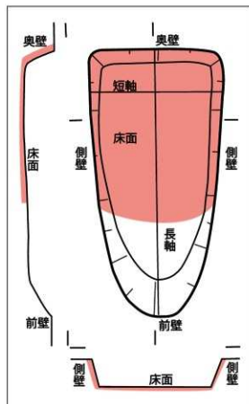
土師器焼成坑構造図
