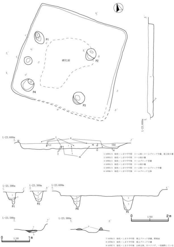
第 62 図 第 15 号壁穴建物跡 (1)
