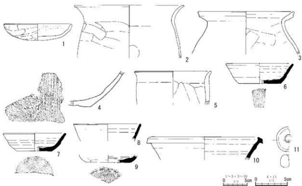
第56图 第10号竖穴建物跡(2)
