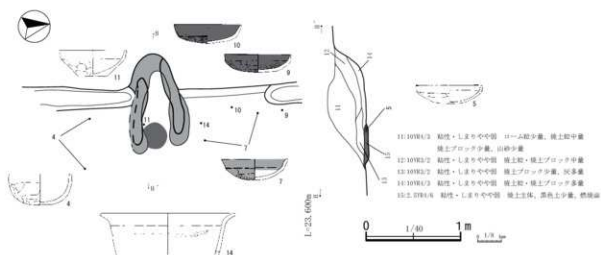
第 37 図 第 11・26 号 竪穴建物跡 (2)
