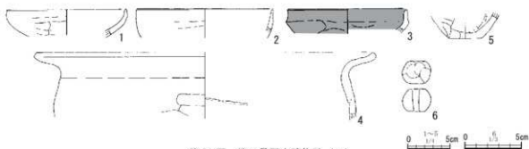
第31図 第6号竪穴建物跡(2)
