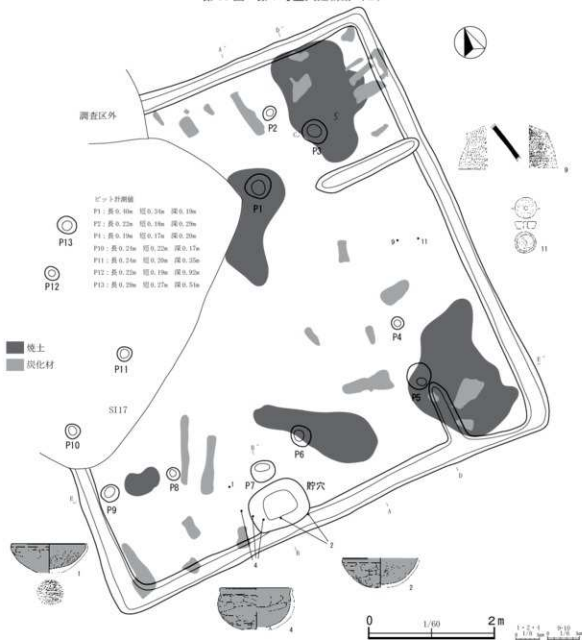
第 34 图 第 9 号竖穴建物跡 (1)
