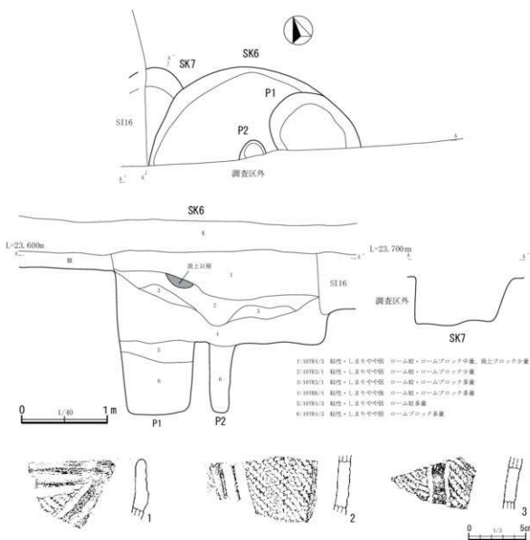
第12図 第5・7号土坑・第6号土坑(1)
