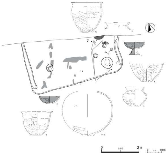
第21図 第3号竪穴建物跡(2)
