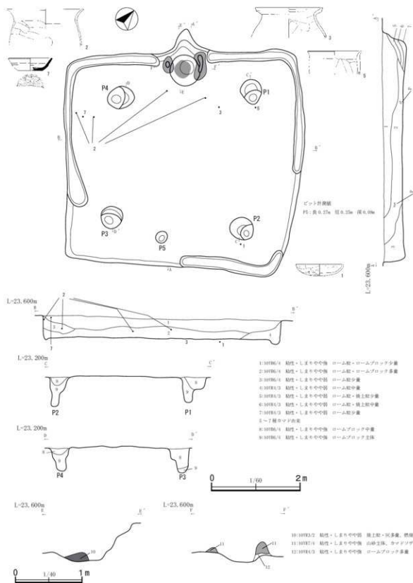
第 55 図 第 10 号竪穴建物跡 (1)
