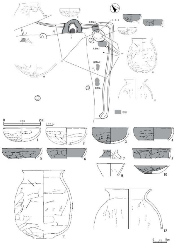
第 44 図 第 23 号竪穴建物跡 (2)
