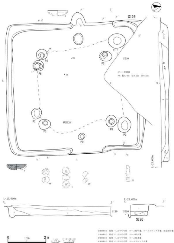
第 36 図 第 11・26 号竪穴建物跡 (1)
