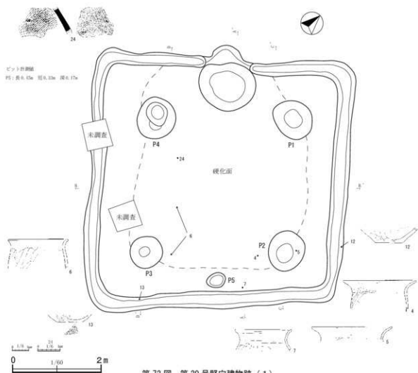
第72図 第20号竪穴建物跡(1)
