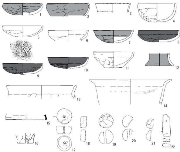
第38図 第11・26号竖穴建物跡(3)
