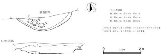
第10図 第21号竪穴建物跡
