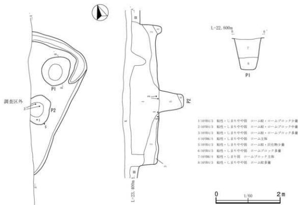
第32図 第7号竪穴建物跡(1)
