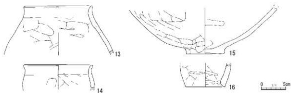
第 45 図 第 23 号竖穴建物跡 (3)
