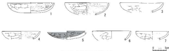
第 59 図 第 12 号竖穴建物跡 (3)
