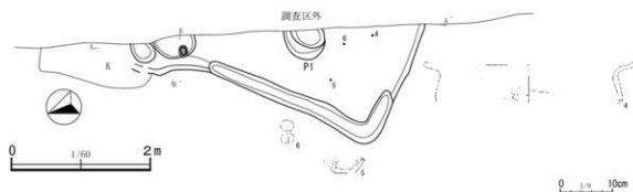
第30图 第6号竖穴建物跡(1)
