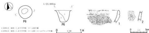
第13図 第6号土坑(2)・第8号土坑・第6号柱穴
