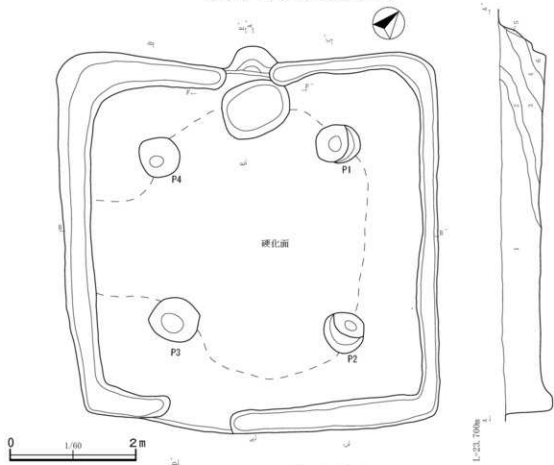
第57图 第12号竖穴建物跡(1)
