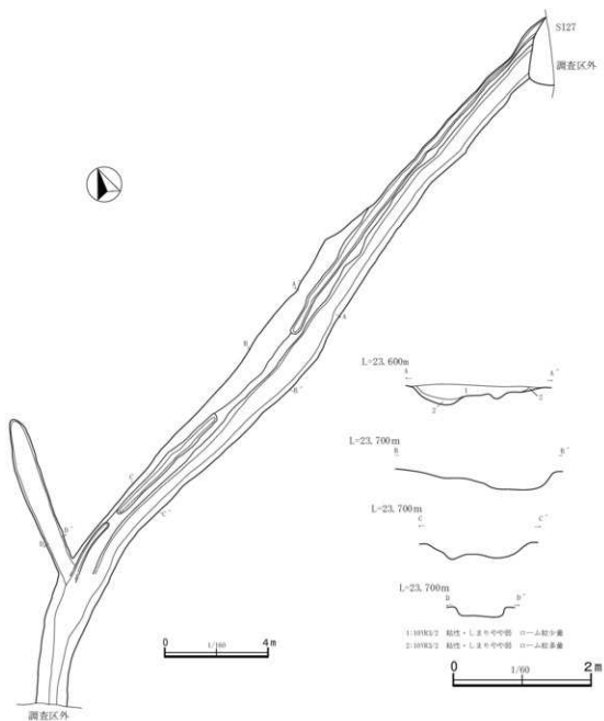
第89図 第2号溝跡
