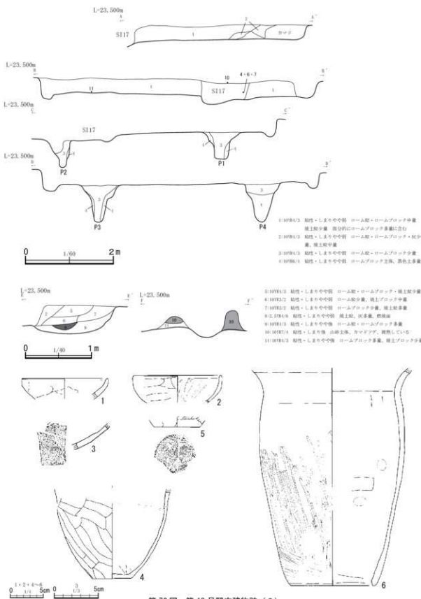
第70図 第18号竪穴建物跡(2)
