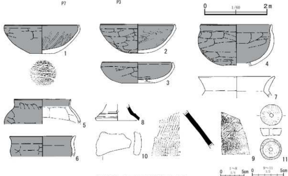
第35図 第9号野穴建物跡(2)
