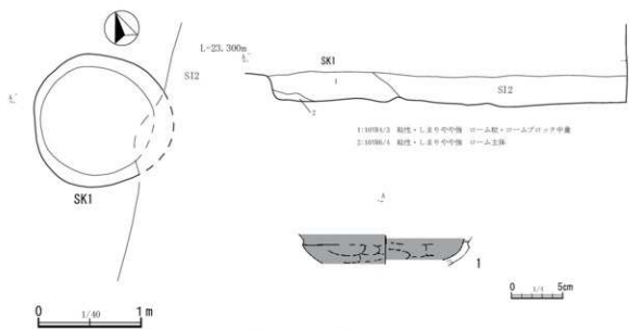
第50図 第1号土坑
