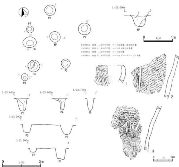
第11図 第28号竪穴建物跡
