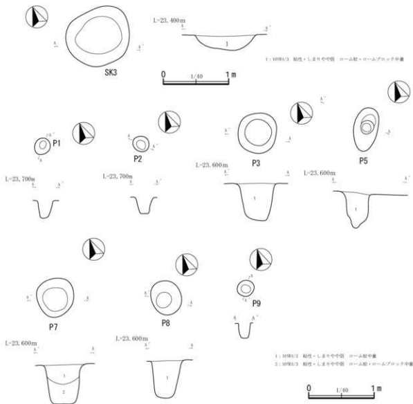
第91図 第3号土坑・第1～3・5・7～9号柱穴
