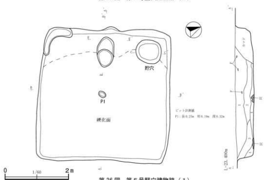
第26図 第5号竪穴建物跡(1)
