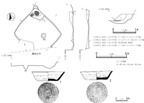
第 61 図 第 13 号竪穴建物跡
