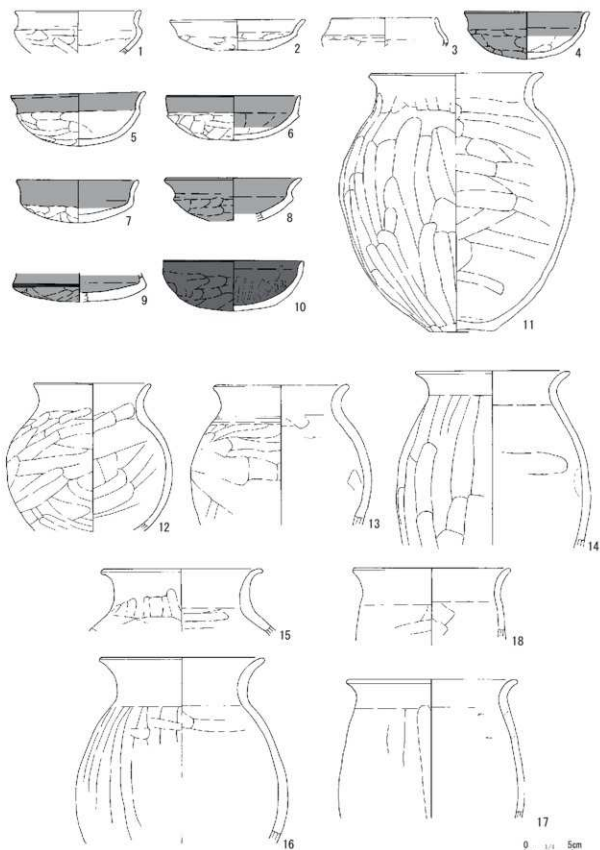
第28圖 第5号竖穴建物跡(3)
