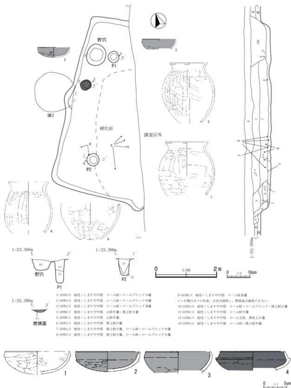
第18図 第2号貯穴建物跡(1)
