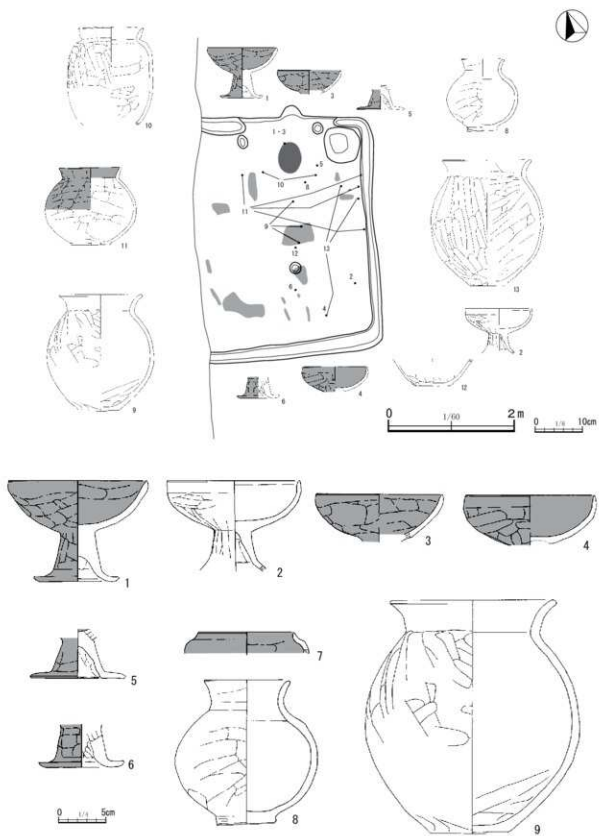
第 24 图 第 4 号竖穴建物跡 (2)
