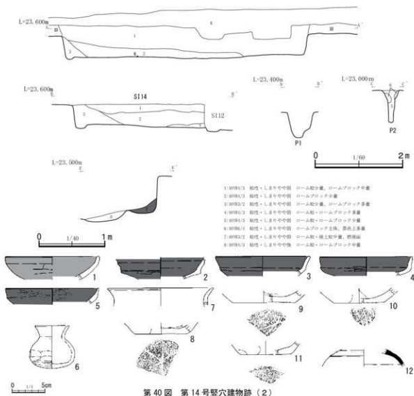
第40図 第14号竪穴建物跡(2)
