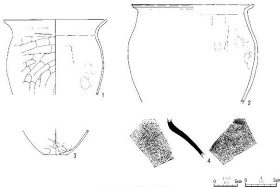
第54図 第8号竪穴建物跡
