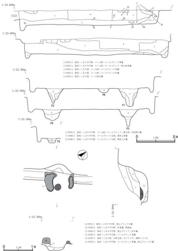
第76図 第22号竪穴建物跡(2)
