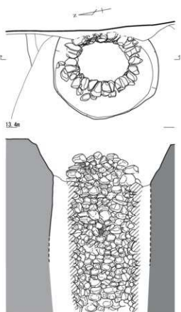
図7 SE1 平・断面図
