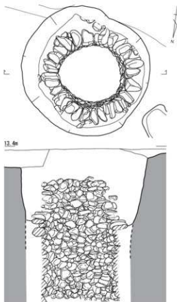
図8 SE3 平・断面図
