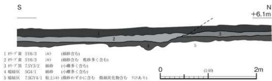
図419 56号墳 断面
