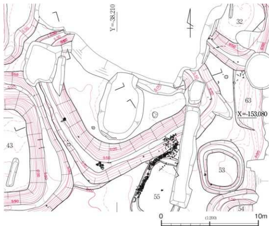
図376 49号墳 平面
