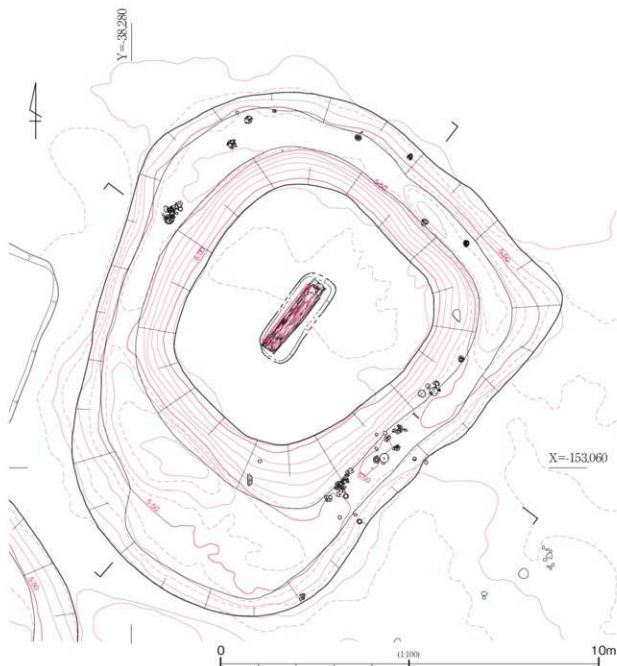
図424 48号墳 平面
