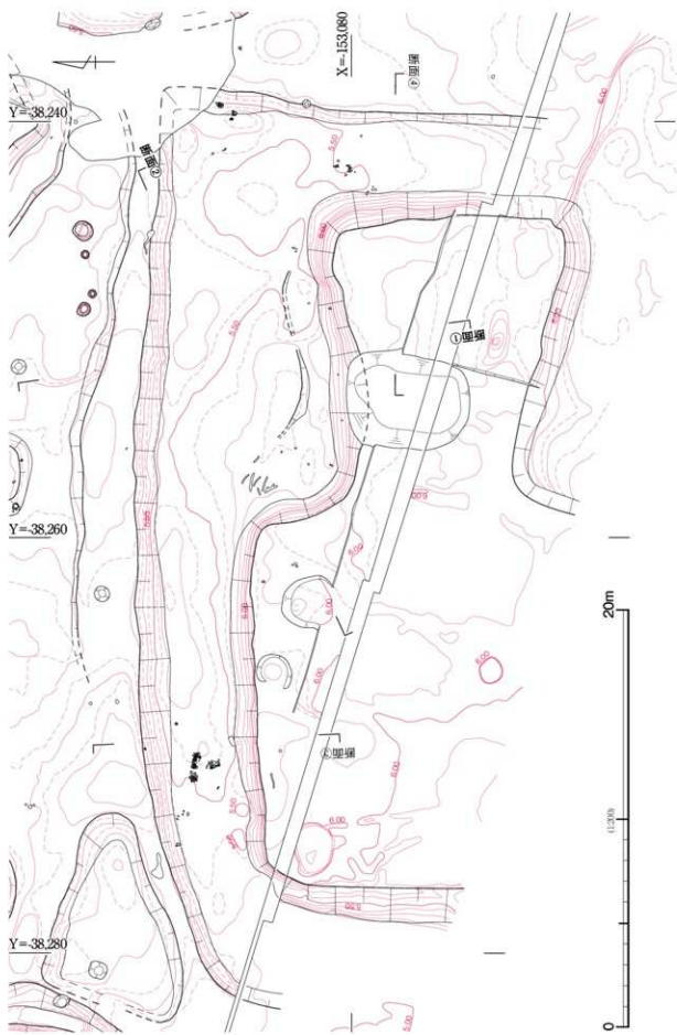
图 436 44号墳 平面
