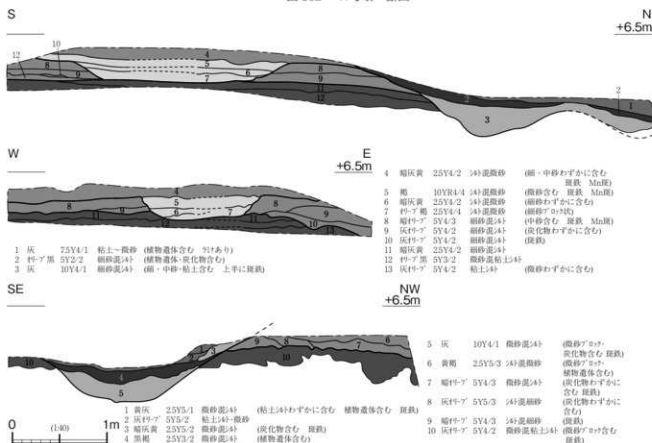
図 363 32号墳 断面
