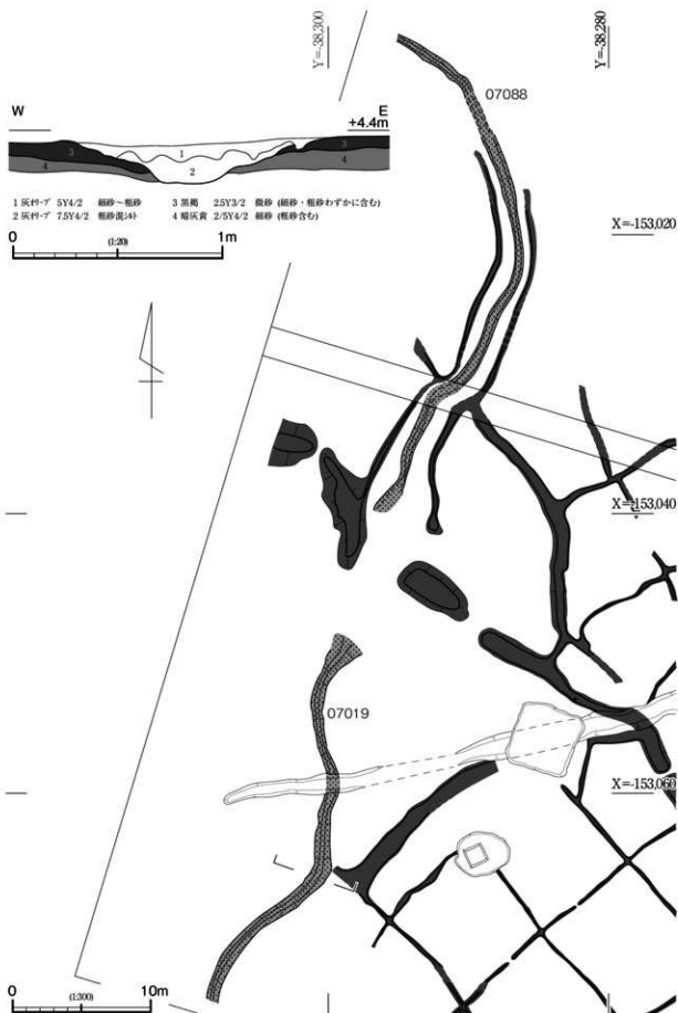
図110 07019溝 平・断面
