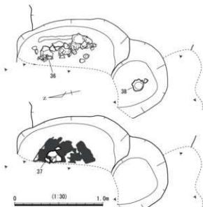
図10 SK8・20 平面図
