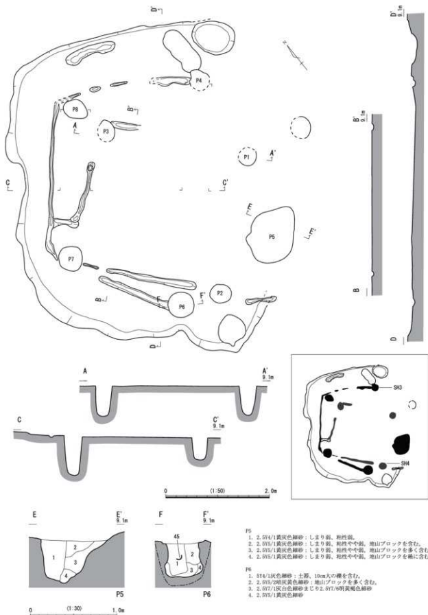
図12 SH3・4 平・断面図
