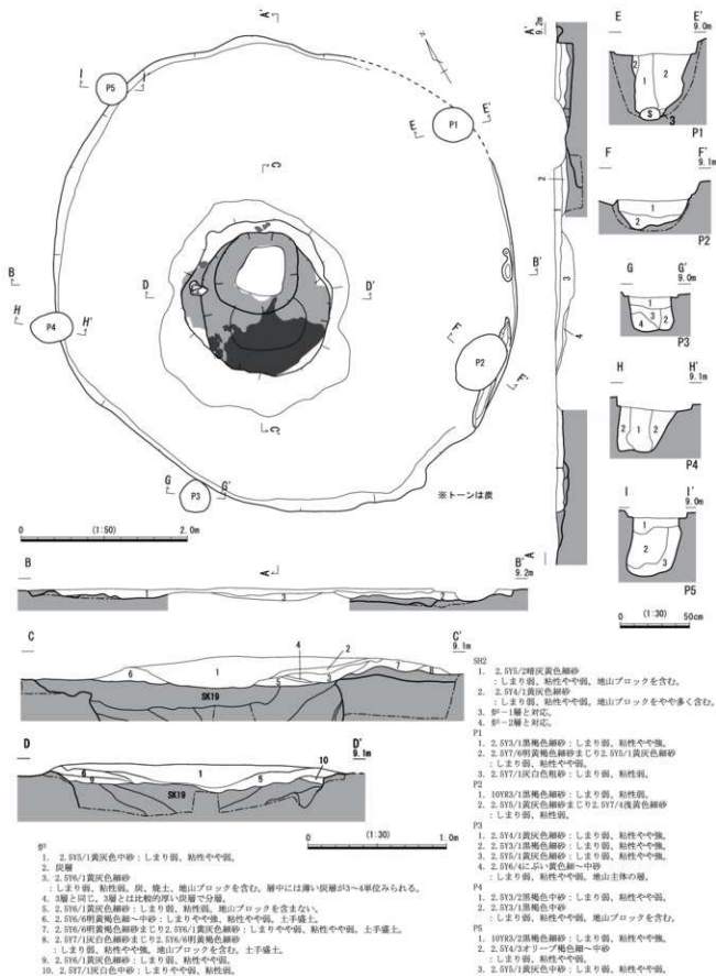
図13 SH2 平・断面図
