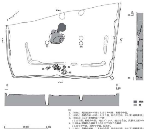
図15 SH1(新) 平・断面図
