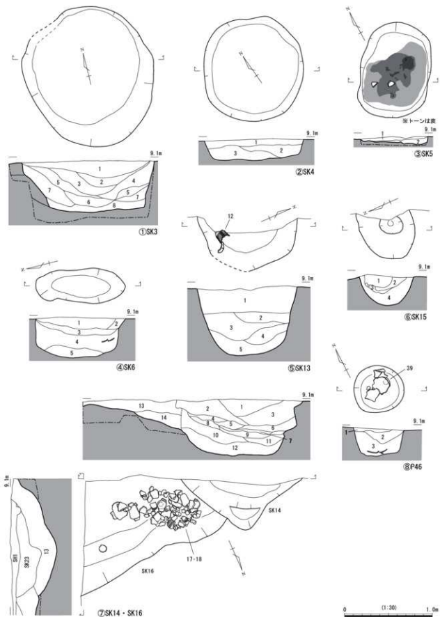
図5 遺構平・断面図
