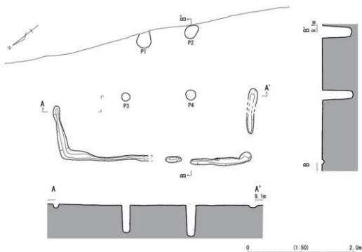
図14 SH1(古) 平・断面図
