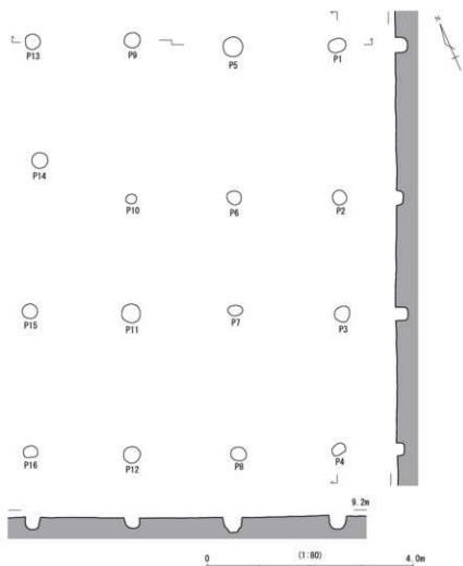
図18 SB1 平・断面図
