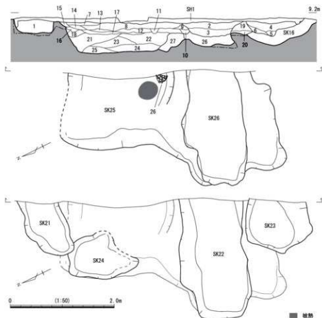
図6 SK21~26 平・断面図
