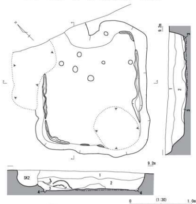
図7 SH6 炭・焼土検出状況平・立面図
