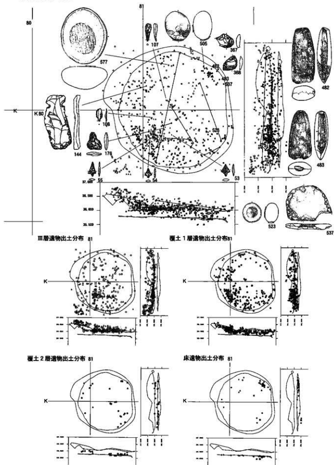
図81 B・C地区の住居跡(63) A H18(3)
