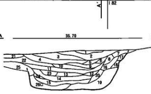
図159 B・C地区の土坑(32) CP 98, 175, 178
