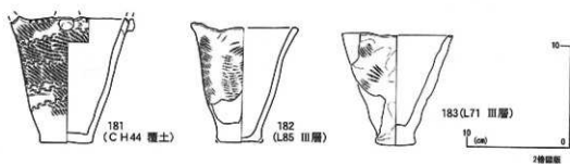
図217 B・C地区出土の土器(33)
