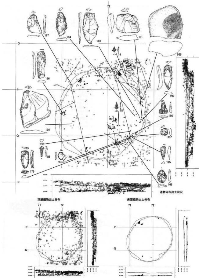
図22 B・C地区の住居跡(4) AH1(3)
