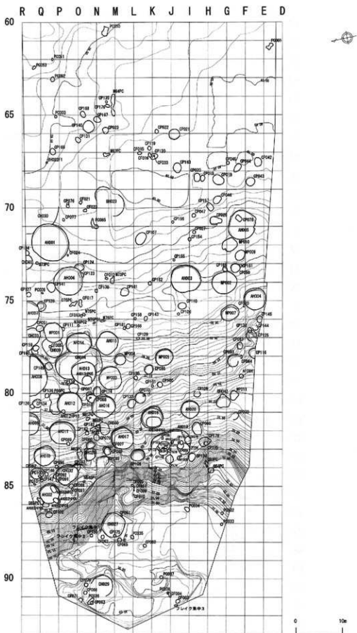
図15 B地区遺構位置図・最終確認面地形図
