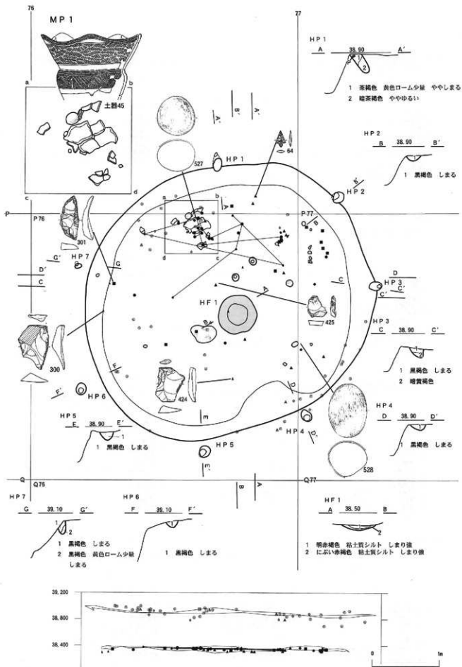
図117 B・C地区の住居跡(99) MP 1(1)
