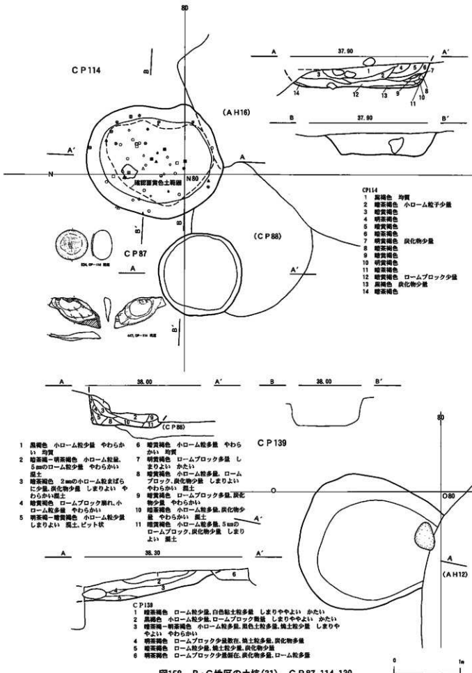
図158 B・C地区の土坑(31) CP87、114、139
