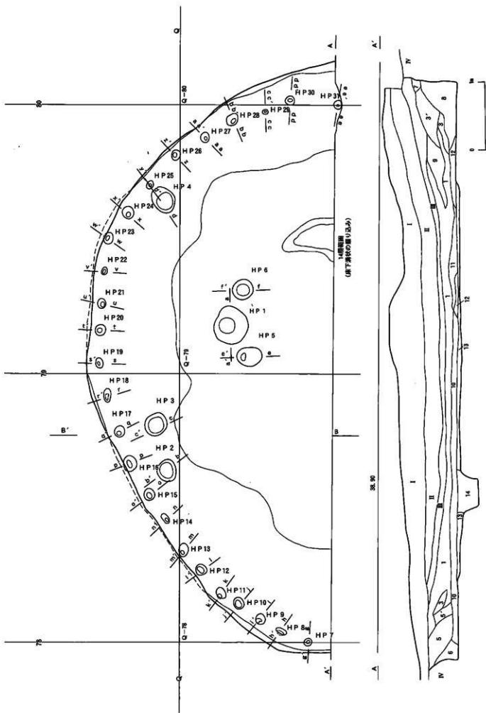
図46 B・C地区の住居跡(28) AH8(1)
