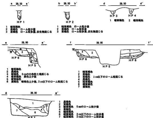
図67 B・C地区の住居跡(49) A H14(2)
