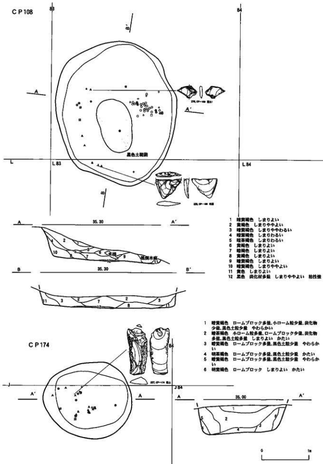
図164 B・C地区の土坑(37) CP 108, 174
