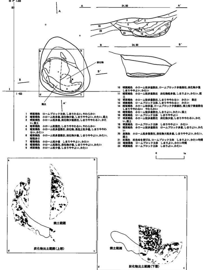
図161 B・C地区の土坑(34) B P 138
