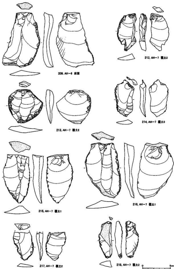
図235 B・C地区遺構出土の石器(14)
