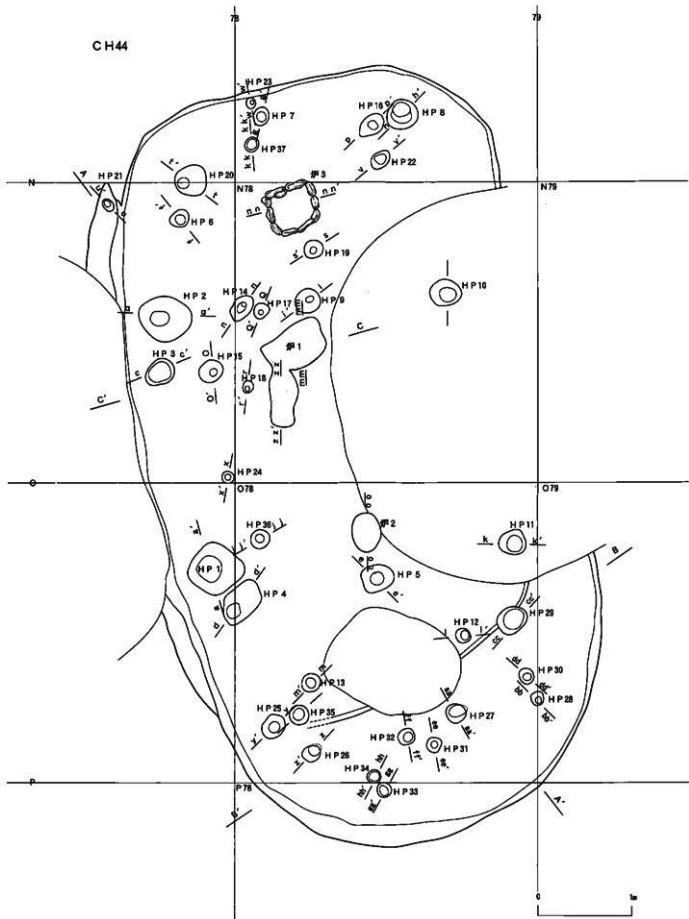
図111 B・C地区の住居跡(93) CH44(1)
