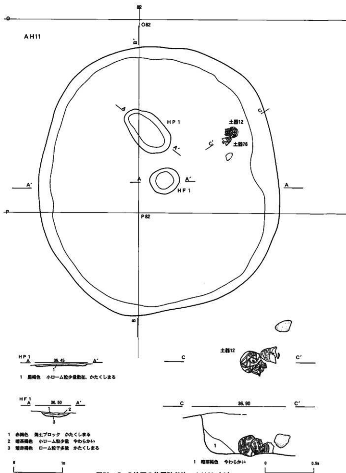
図56 B・C地区の住居跡(38) AH11 (1)
