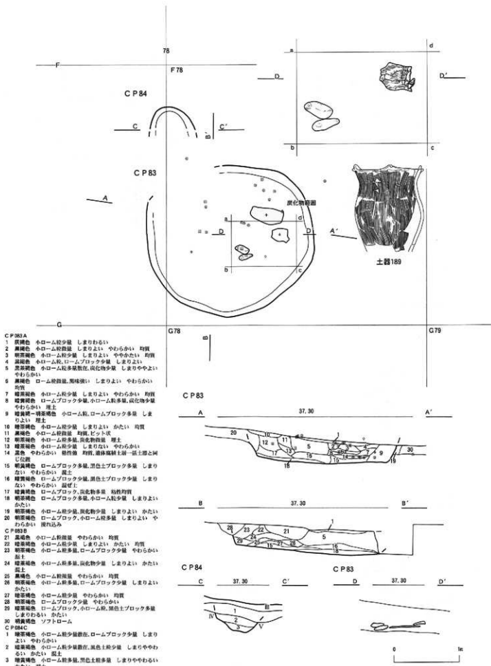
図151 B・C地区の土坑(24) CP83, 84
