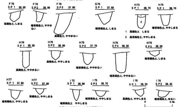
図173 B・C地区の土坑(46) 小ピット群
