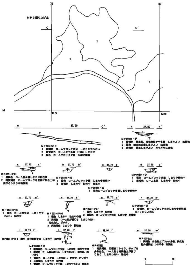
図122 B・C地区の住居跡(104) MP 3(2)
