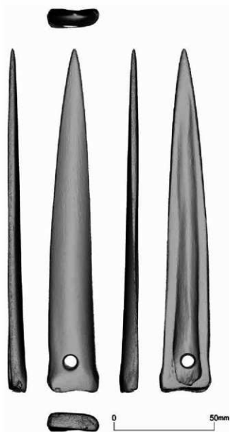
図10 骨角器展開図（陰影図像）
