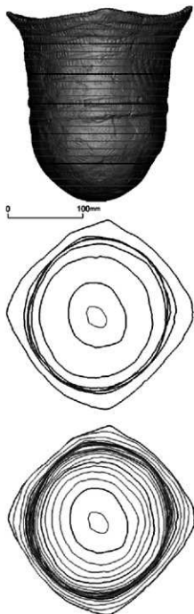
図11 土器連続横断面図
