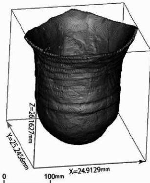
図5 土器の座標系と大きさ
