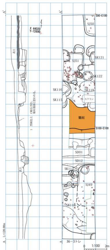
第25図 南辺築垣平面・断面図
