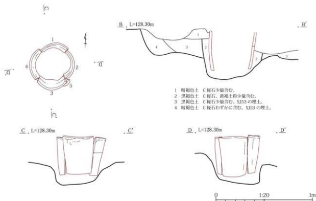
第 21 図 瓦組遺構平面・断面・立面図
