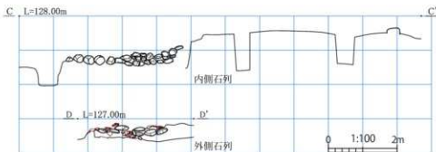
第19図 南大門石列立面図
