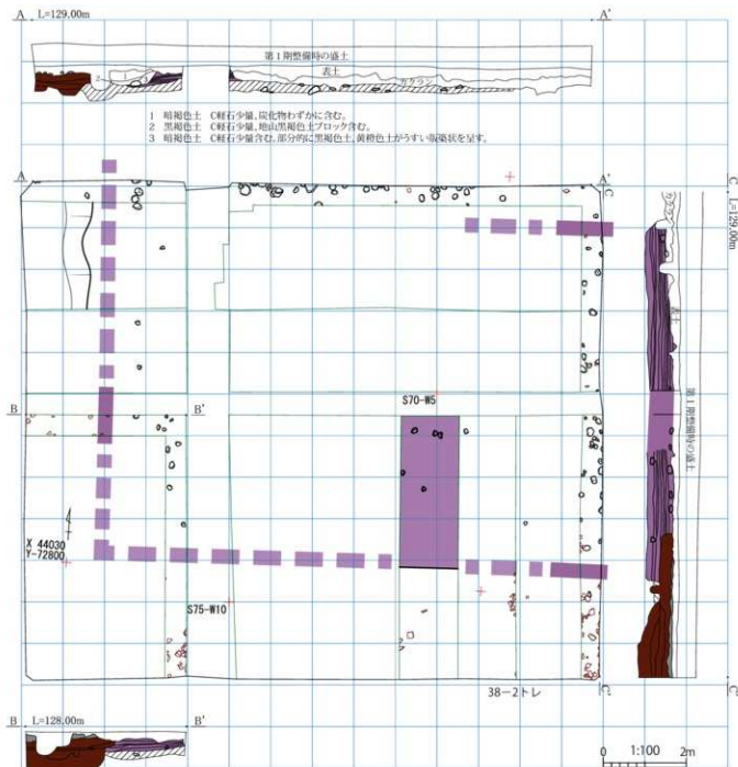
第 12 図 回廊南西角平面・断面図
