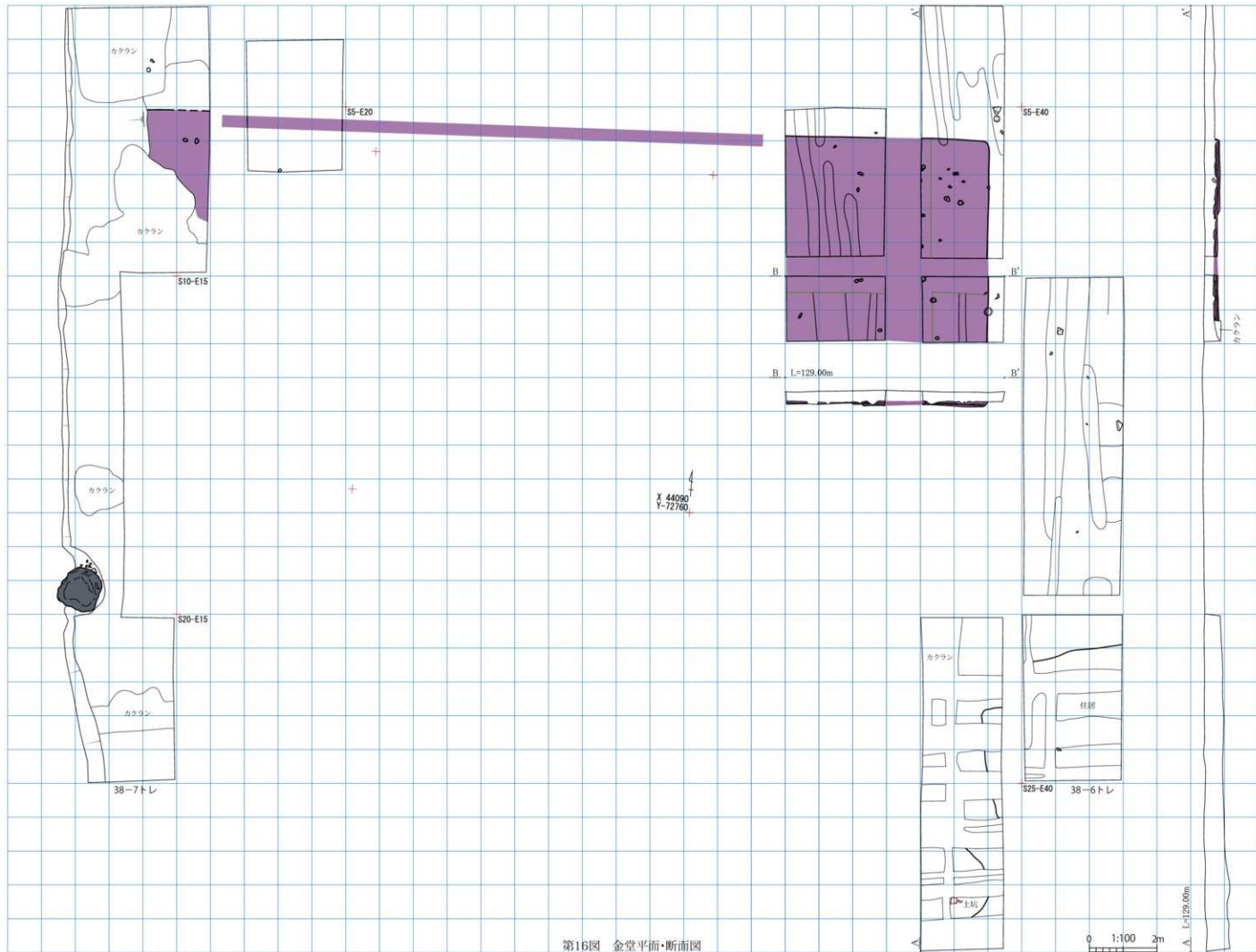
第16図 金堂平面・断面図
