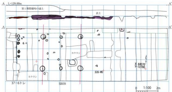
第13図 西面回廊平面・断面図
