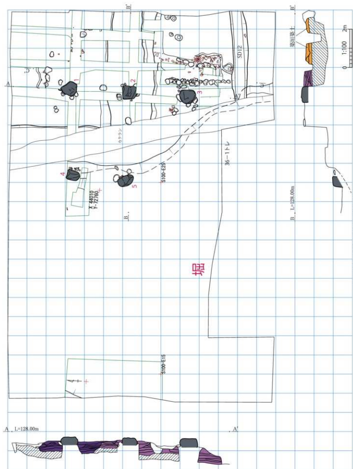
第18図 南大門平面・断面図
