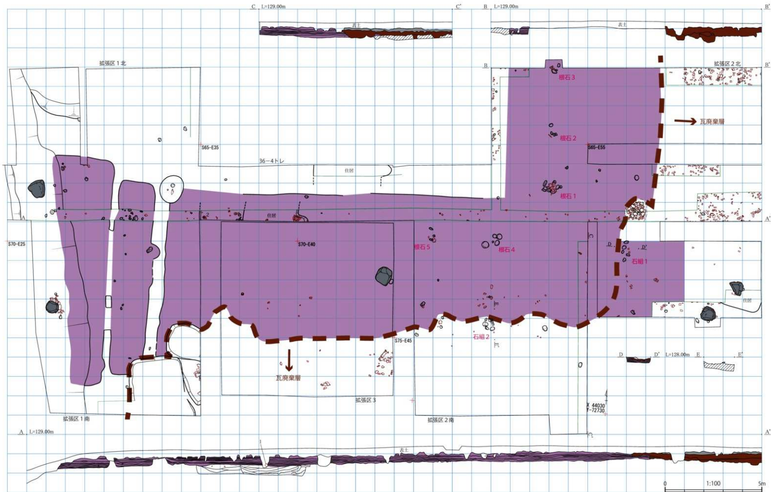
第8图 南面回廊東平面・断面图
