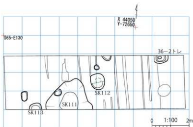
第 26 図 東辺築垣部平面図
