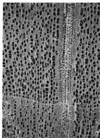
2a. ハノノキ属 (横断面) NEB-5号窯 灰層 bar: 0.5mm
