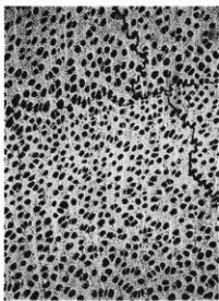
6a.ハインキ属 (横断面) NEB-5号窯 灰層 bar : 0.5mm
