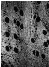
4a.クスギ節 (横断面) NEB-6号窯 bar : 1.0mm
