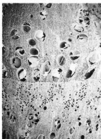
5a.クリ (横断面) NEB-5号窯 灰層 bar : 1.0mm
