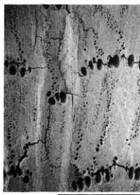
3a. コナラ (横断面) NEB-5号窯 SKI bar: 0.5mm
