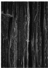
6b.同 (接線断面) bar : 0.1mm
