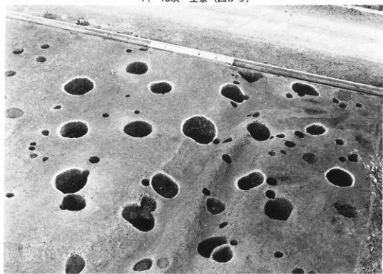
2. 10次 SB-1 (西から)
