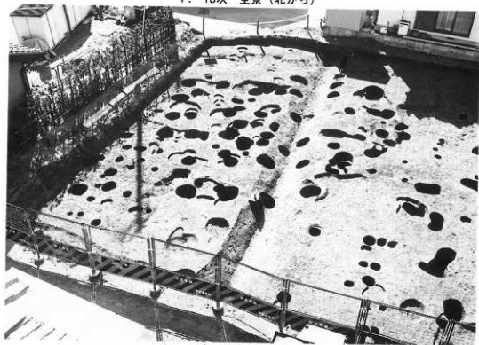
2. 13次 東半全景 (北から)
