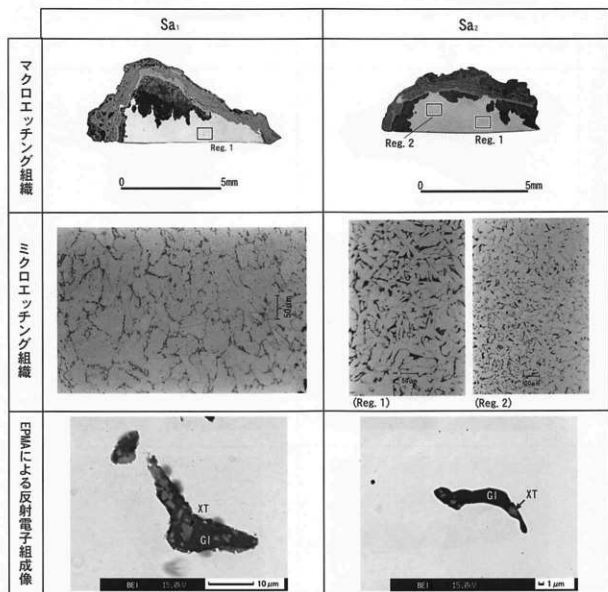
図3 No. 3から抽出した試料の組織観察結果 組織観察用試料は外観の矢印を付した部分から抽出。マイクロエッチング組織はマクロエッチング組織領域(Reg. 1)または領域(Reg. 2)内部。エッチングはナイトールによる。XT=鉄チタン酸化物、GI=ガラス質ケイ酸塩。
